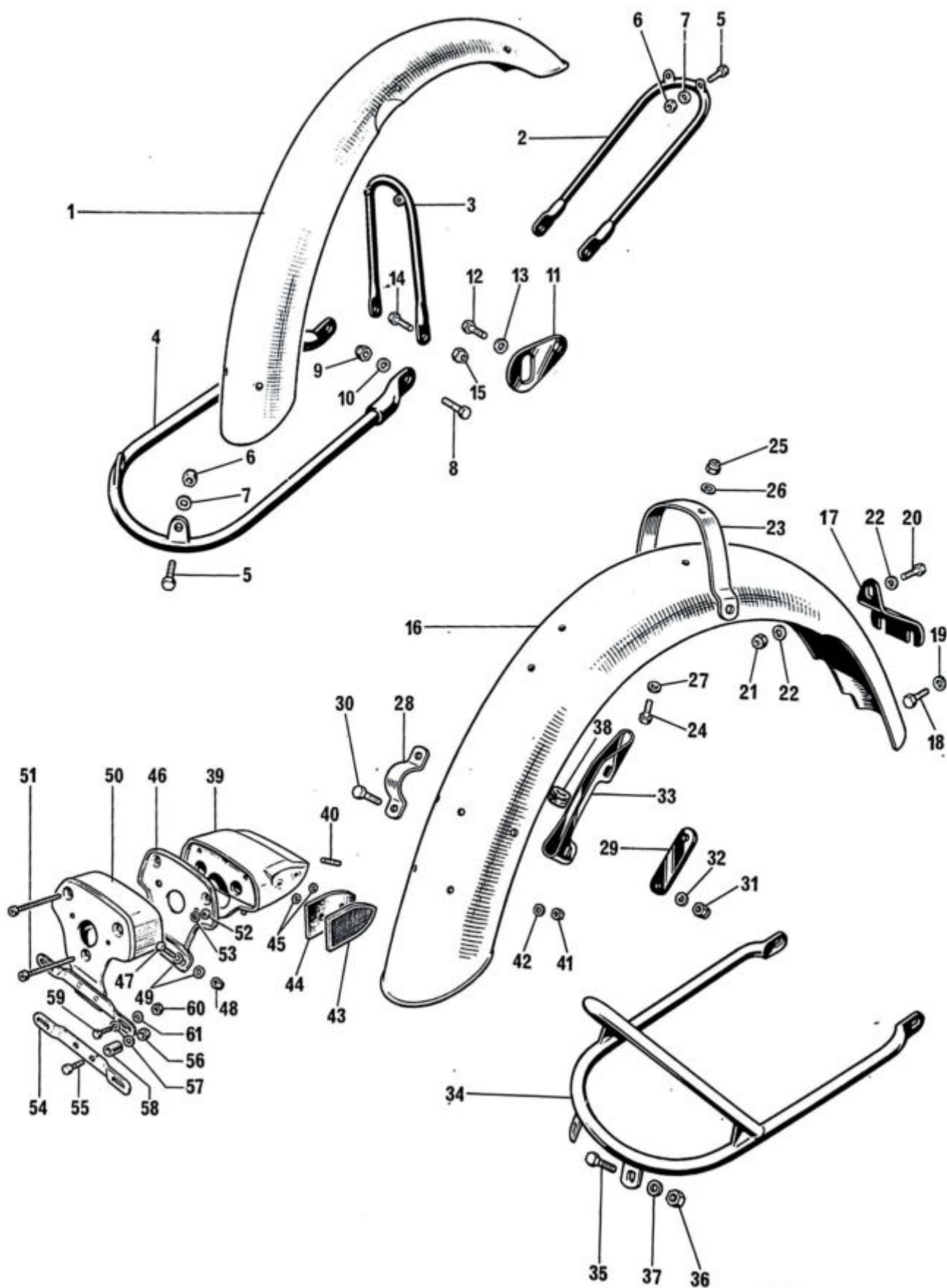
Fig. 28. MUDGUARDS (FENDERS)
