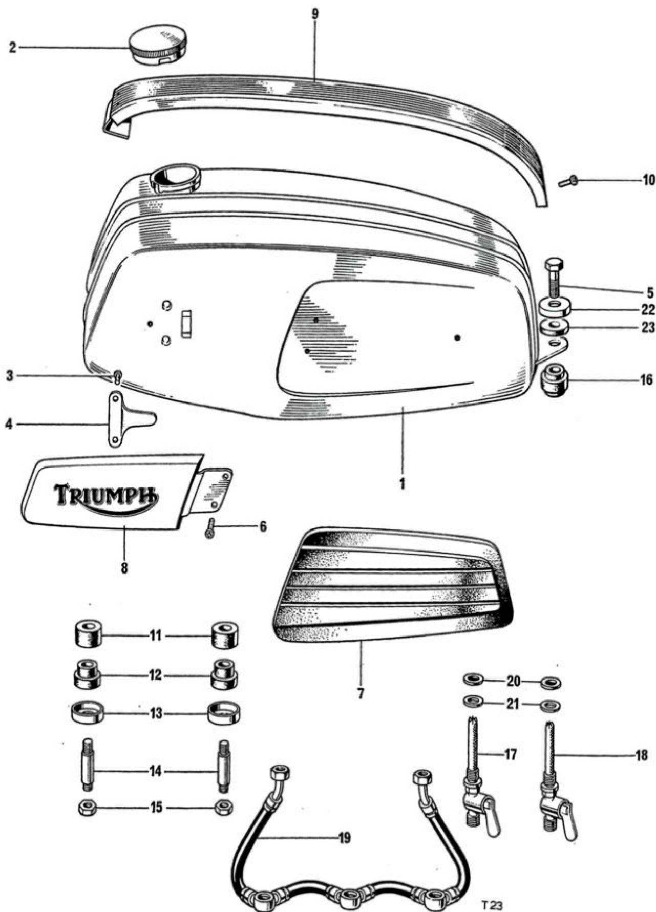
Fig. 23. PETROL (GAS) TANK
