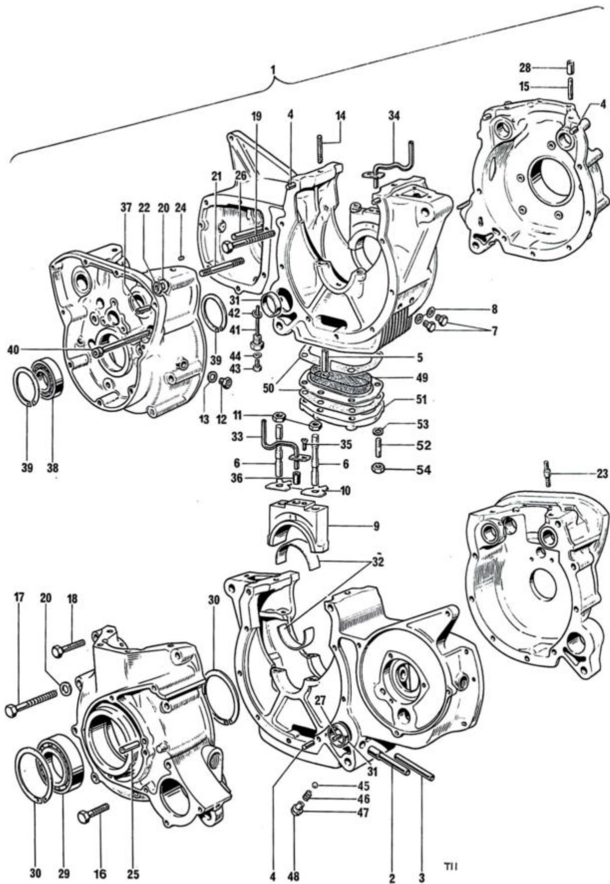
Fig. 2. CRANKCASES
