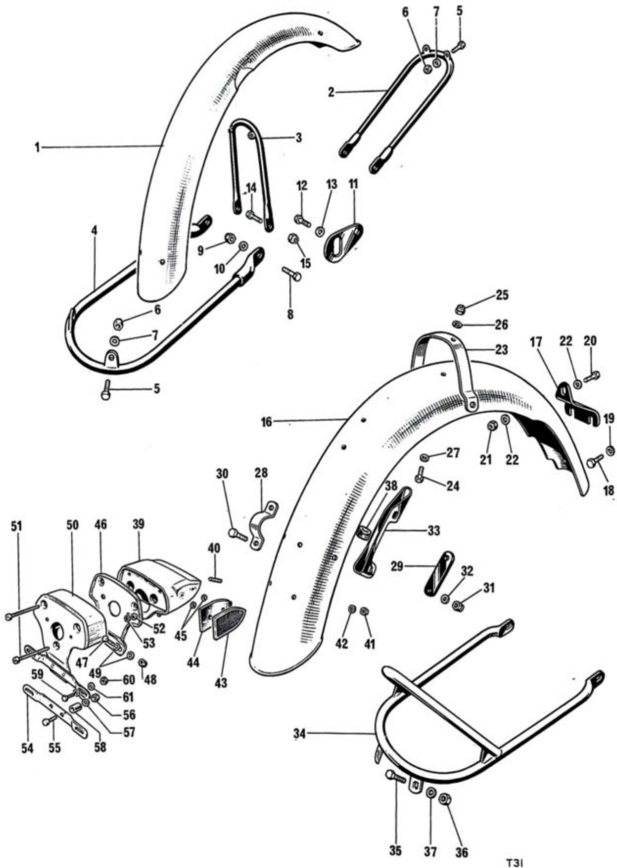
Fig. 27. MUDGUARDS (FENDERS)
