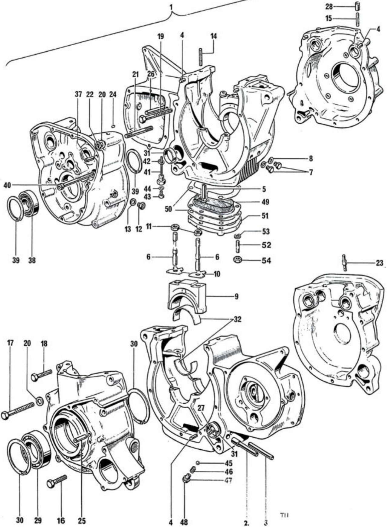
Fig. 2. CRANKCASES
