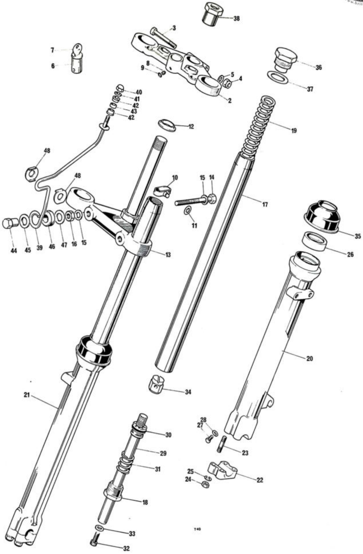
Fig. 20. TELESCOPIC FRONT FORK
