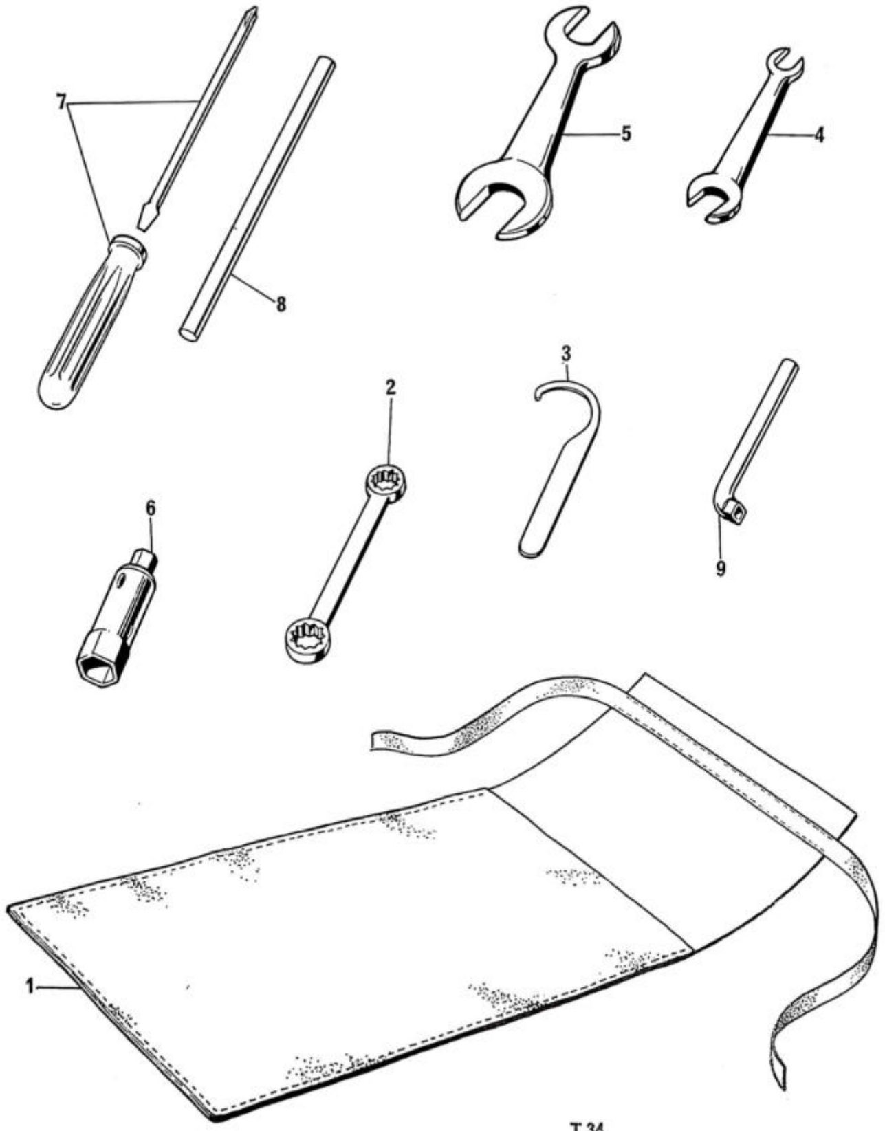
Fig. 32. TOOLKIT
