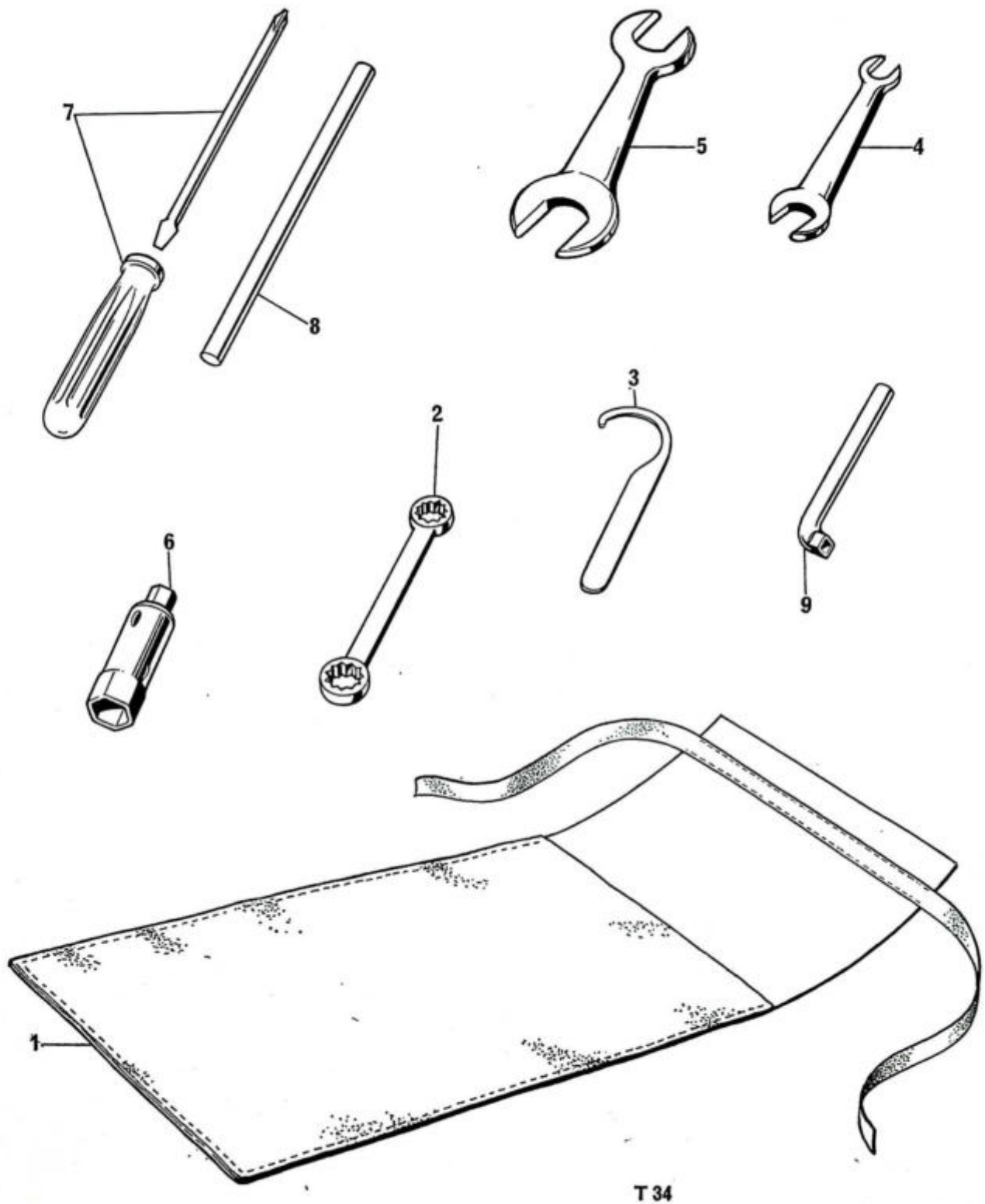
Fig. 32. TOOLKIT
