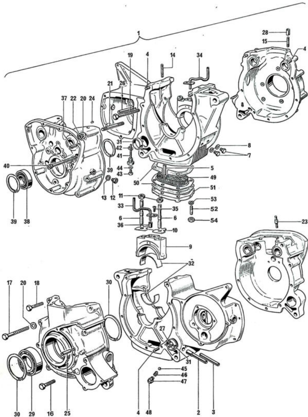
Fig. 2. CRANKCASES
