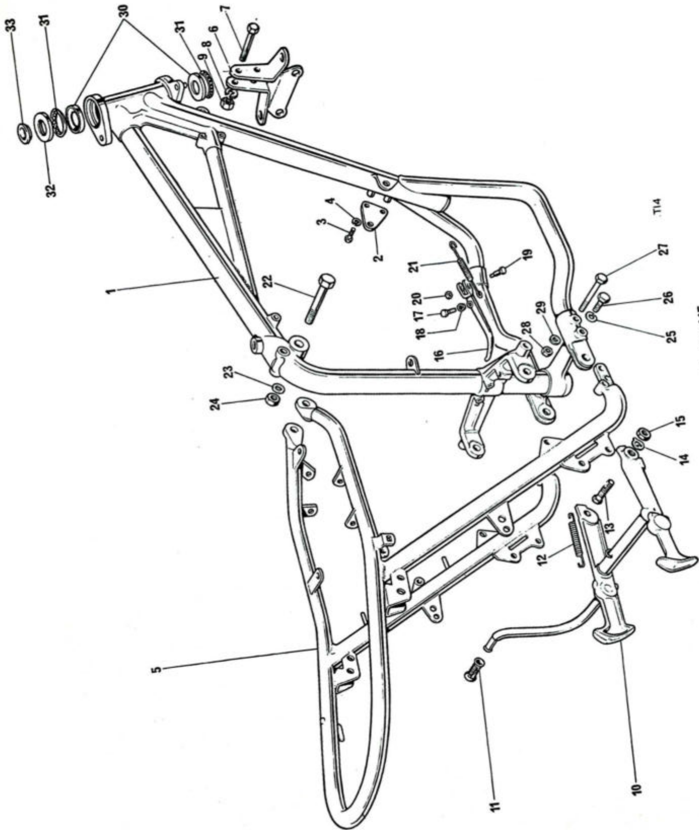
FIG. 16. FRAME
