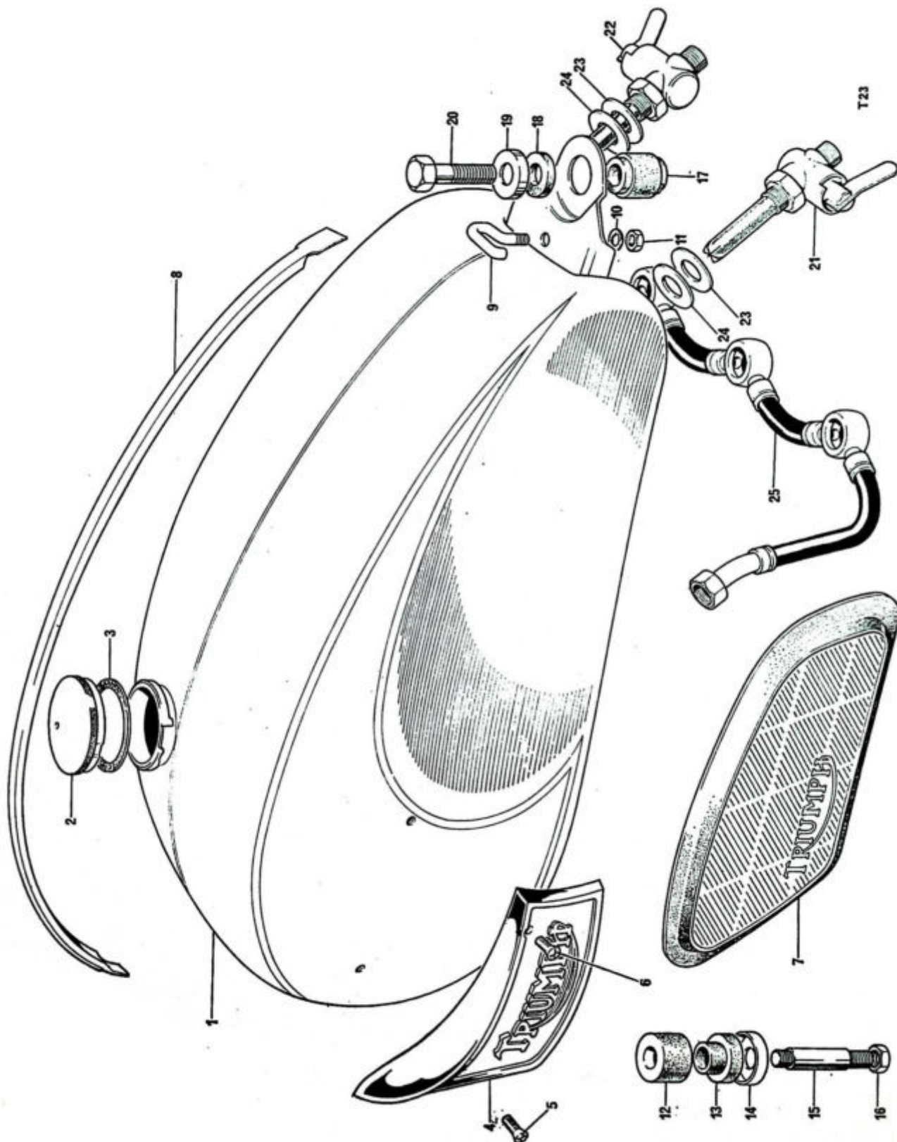
Fig. 25. GAS TANK
