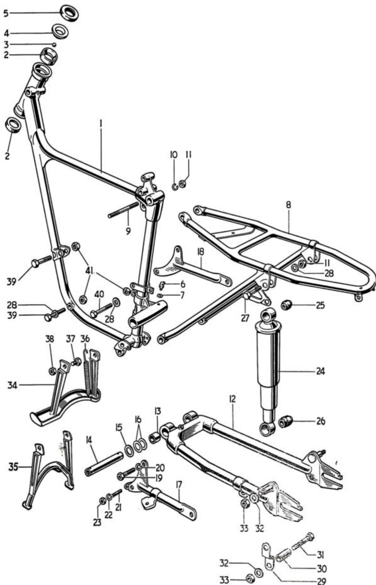
Fig. 7. FRAME COMPLETE
