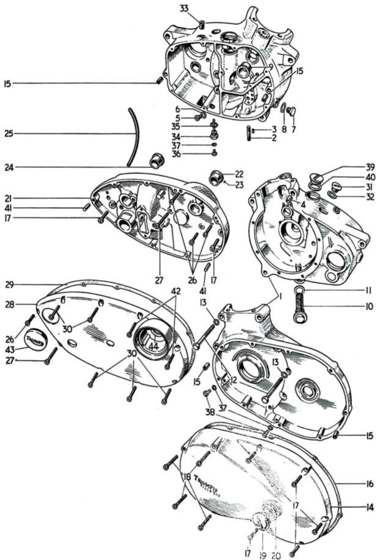
Fig. 2. CRANKCASE
