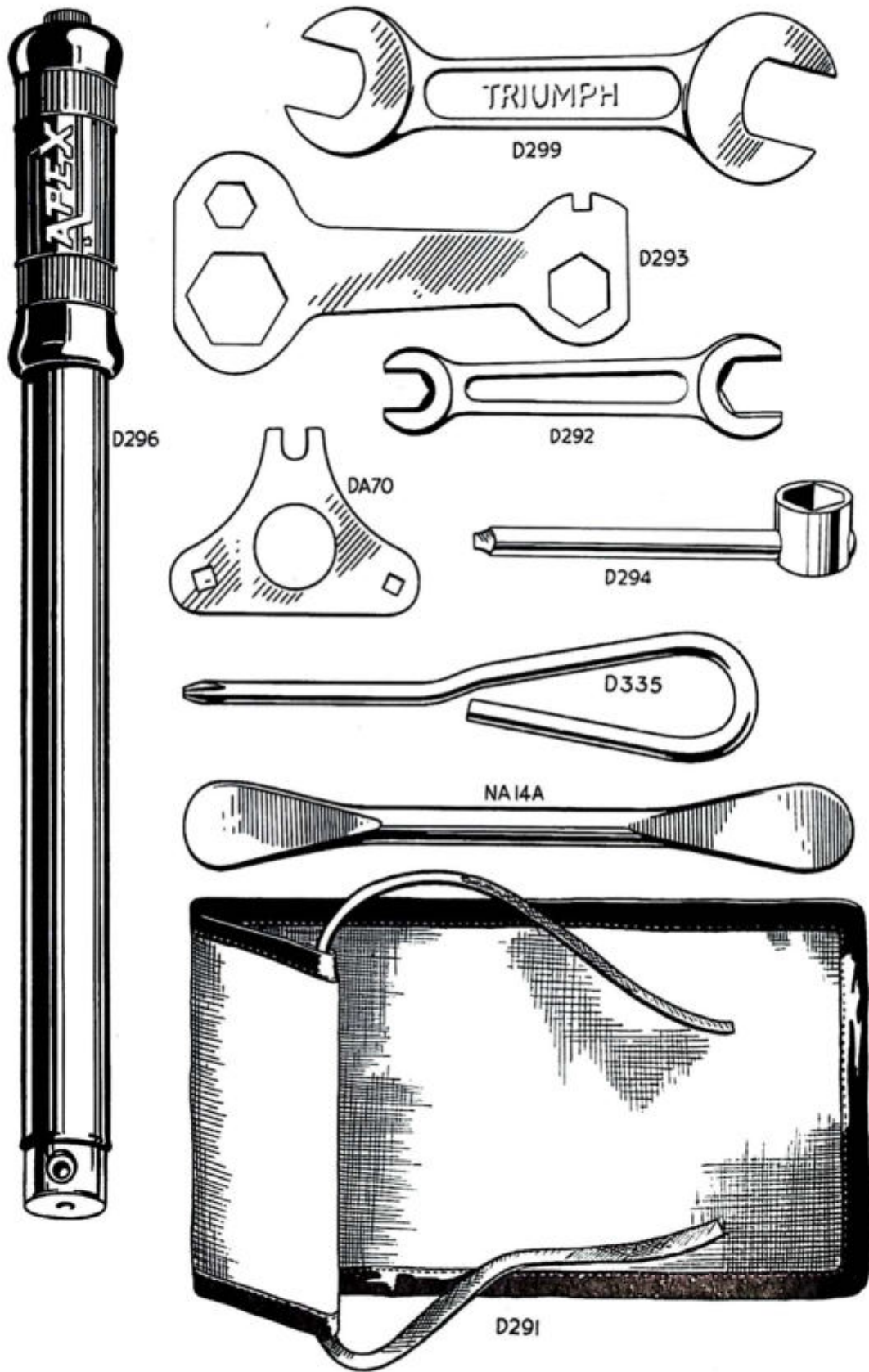
FIG. 12. TOOLS.
