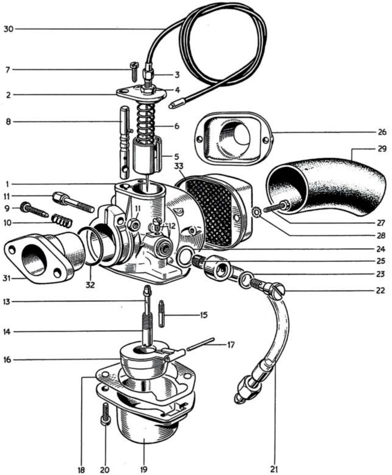
FIG. 15. ZENITH CARBURETTOR
