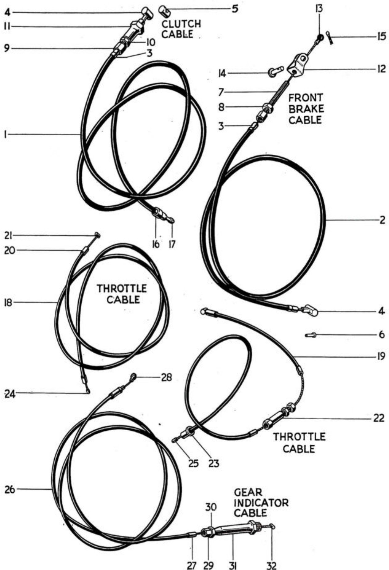
Fig. 23. CONTROL CABLES.
