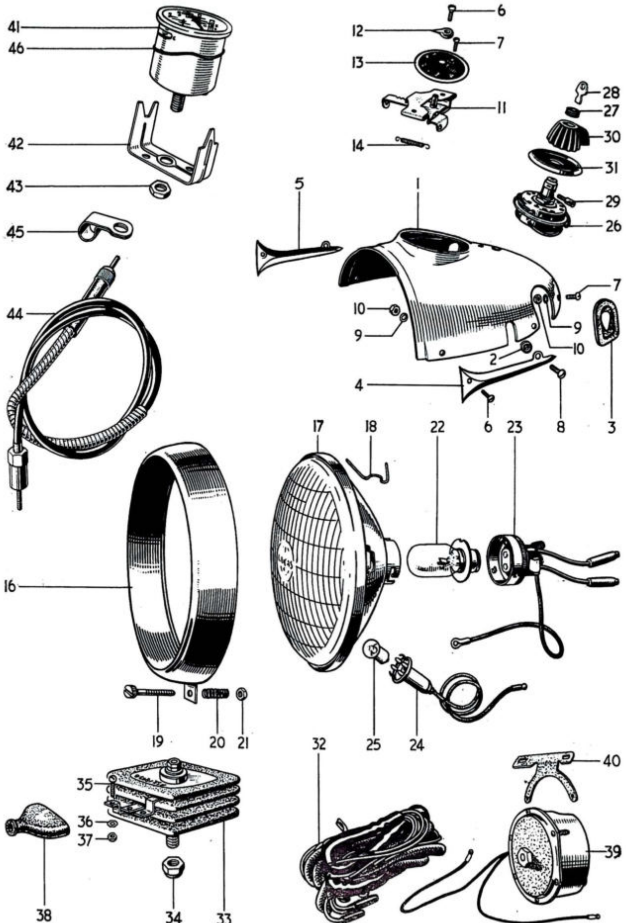
Fig. 12. T20 NACELLE, HEADLAMP, Etc.
