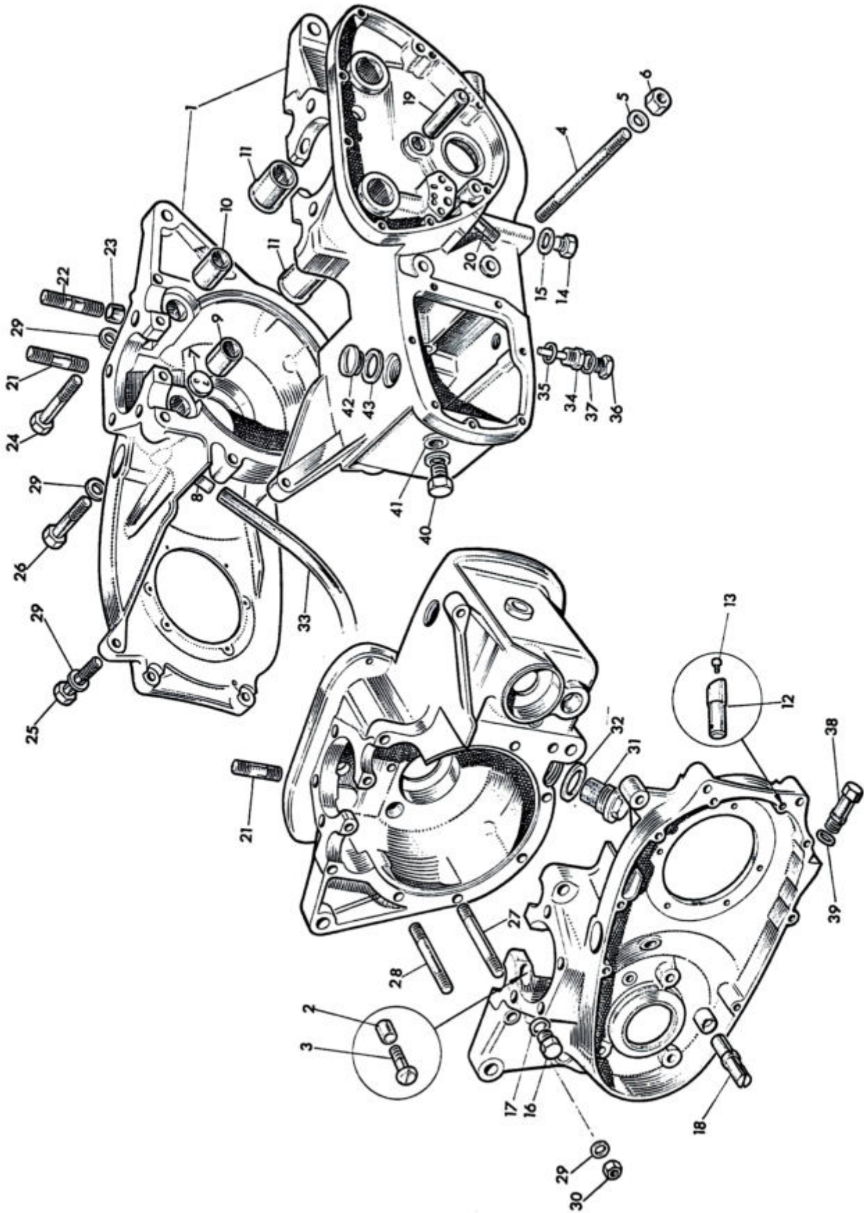
Fig. 2. CRANKCASE
