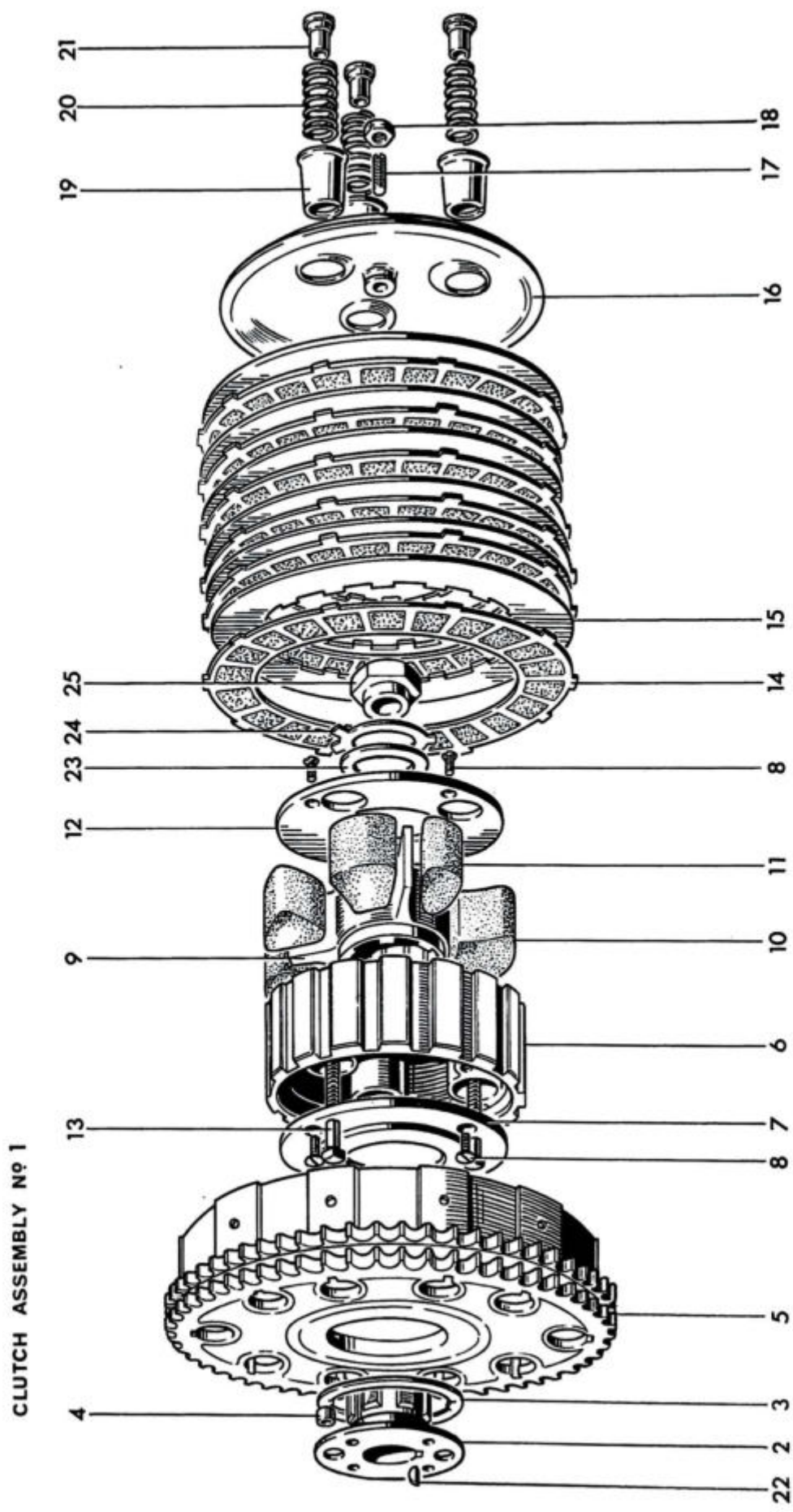
Fig. 10. CLUTCH
