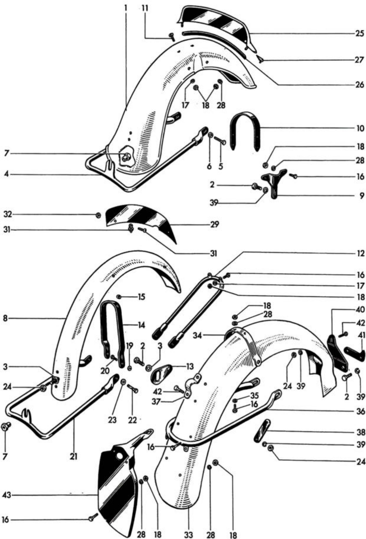
Fig. 26. MUDGUARDS
