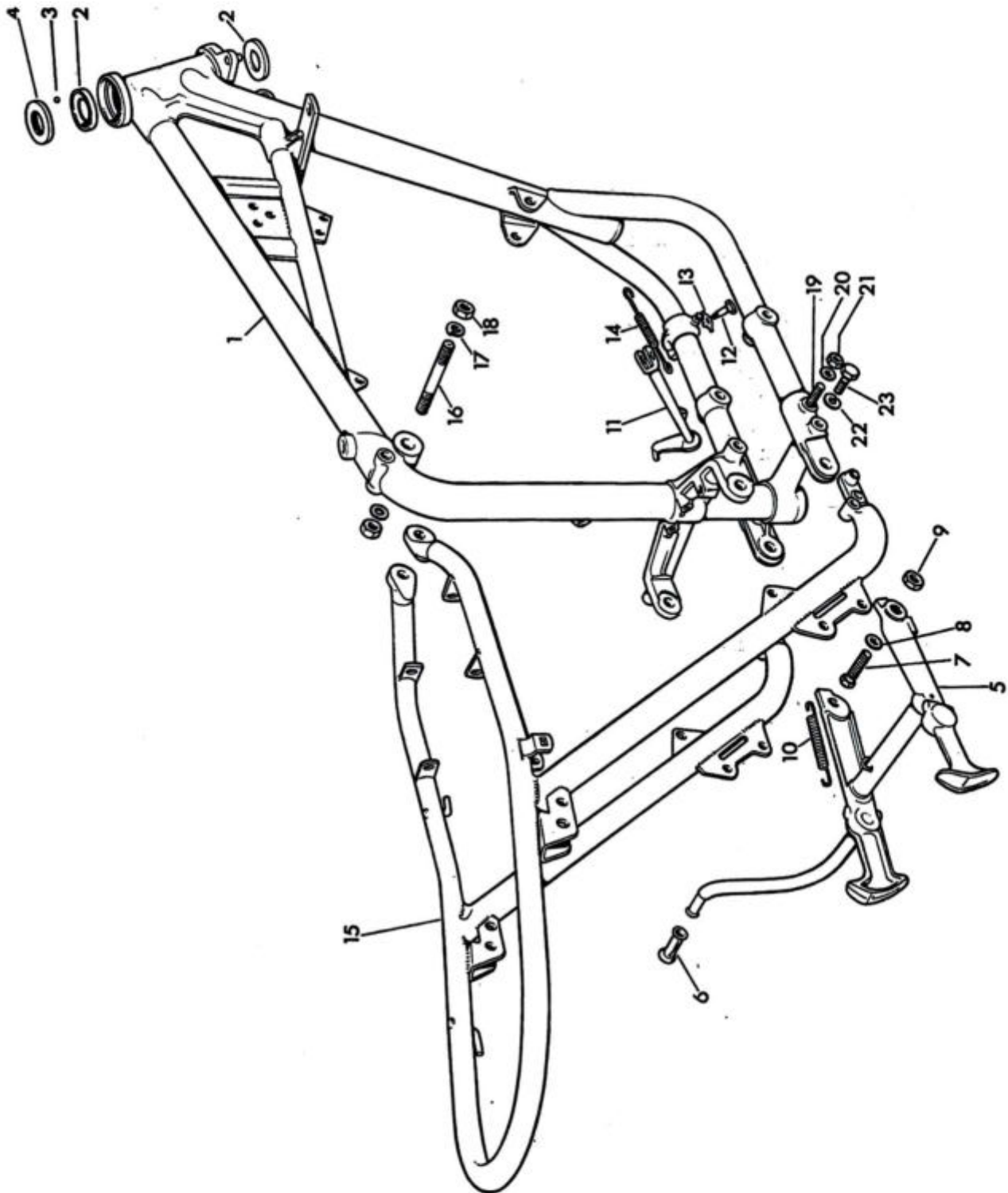
FIG. 12. FRAME
