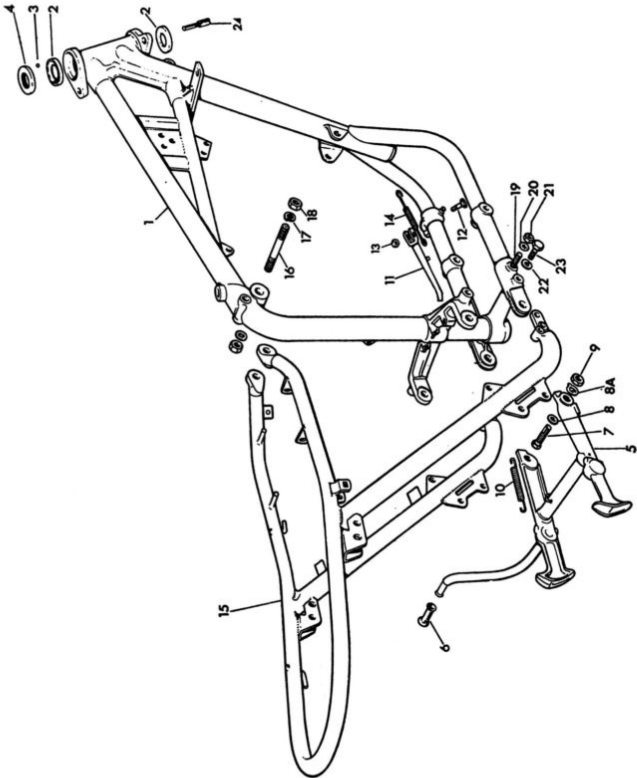
FIG. 12. FRAME
