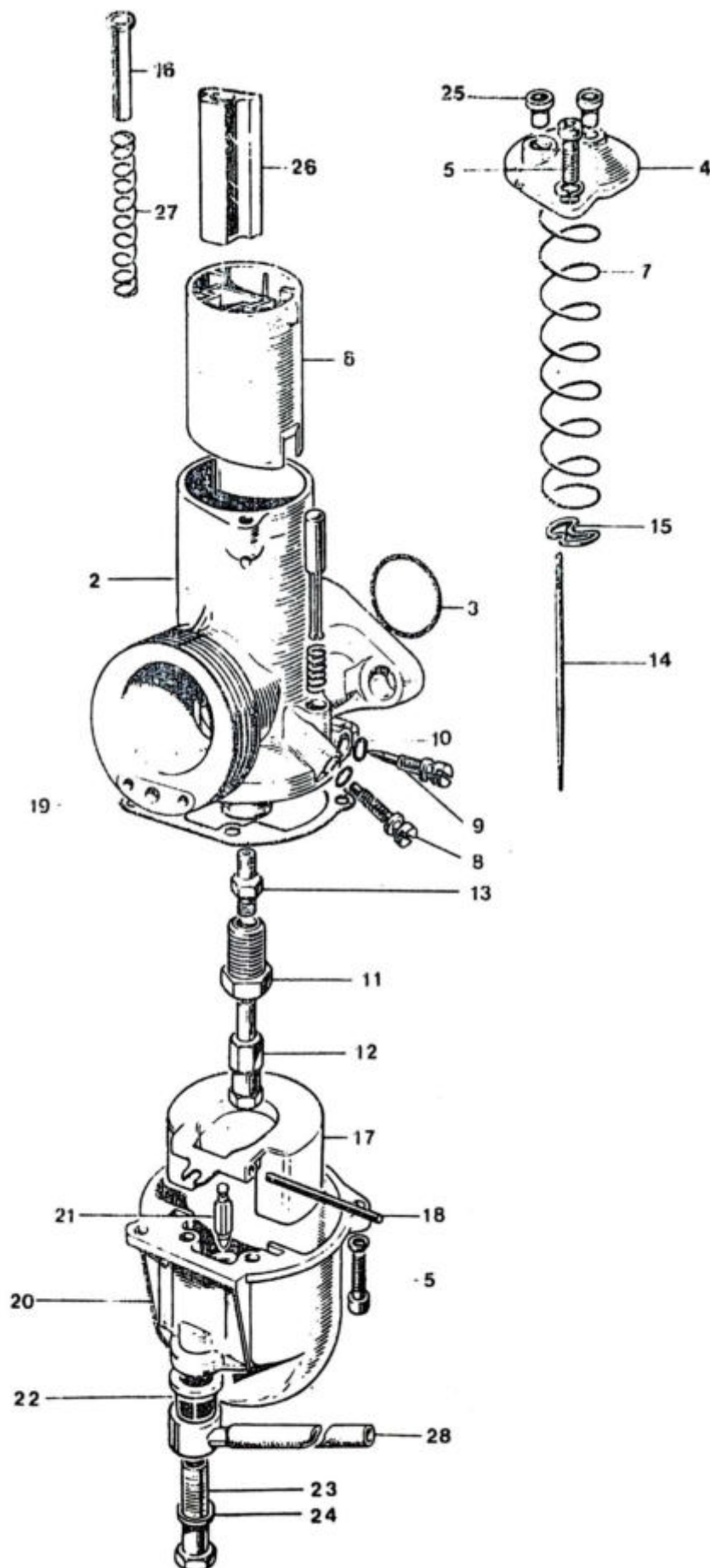
Fig. 29. AMAL CARBURETTER, TR6
