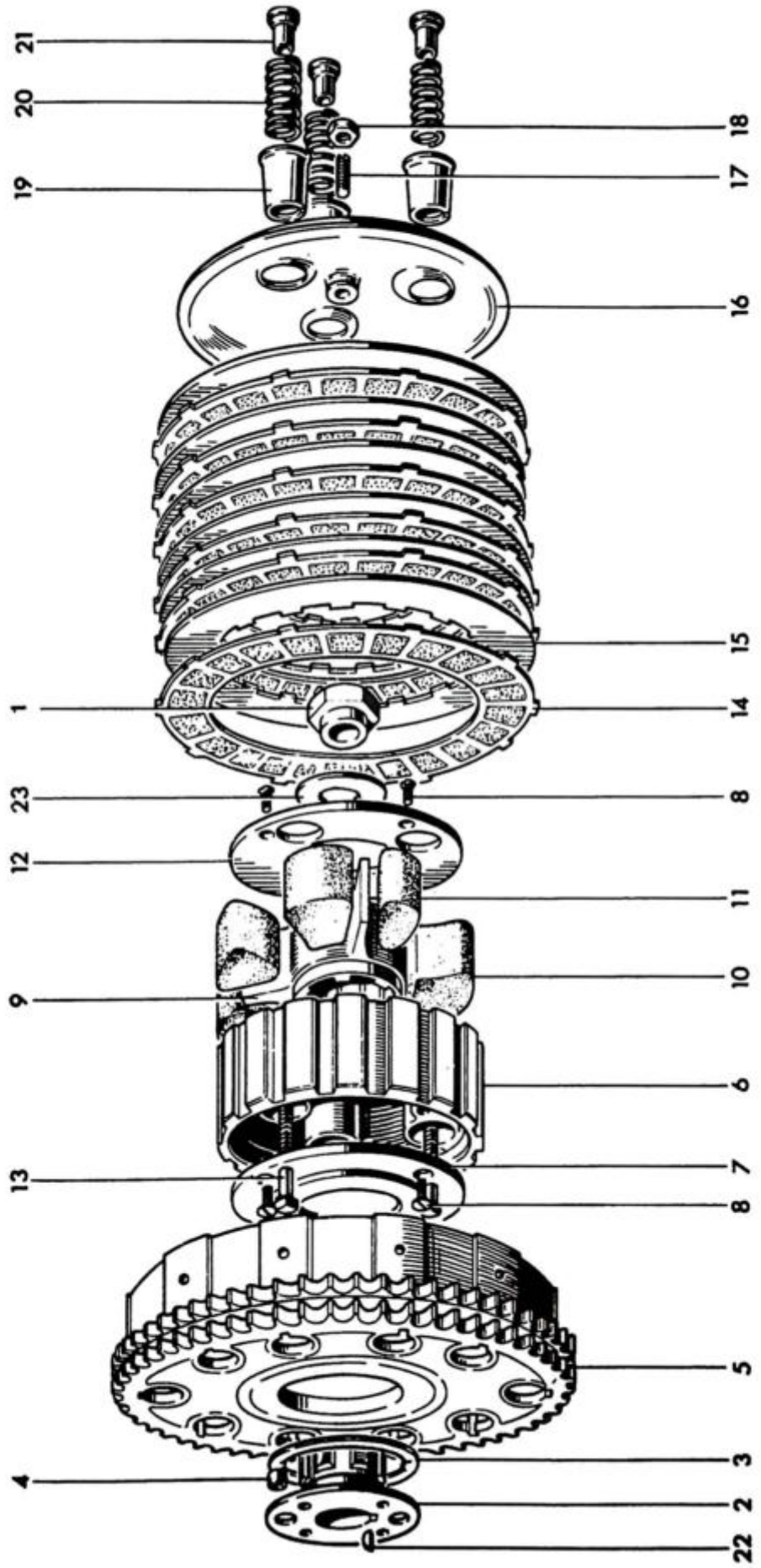
Fig. 10. CLUTCH
