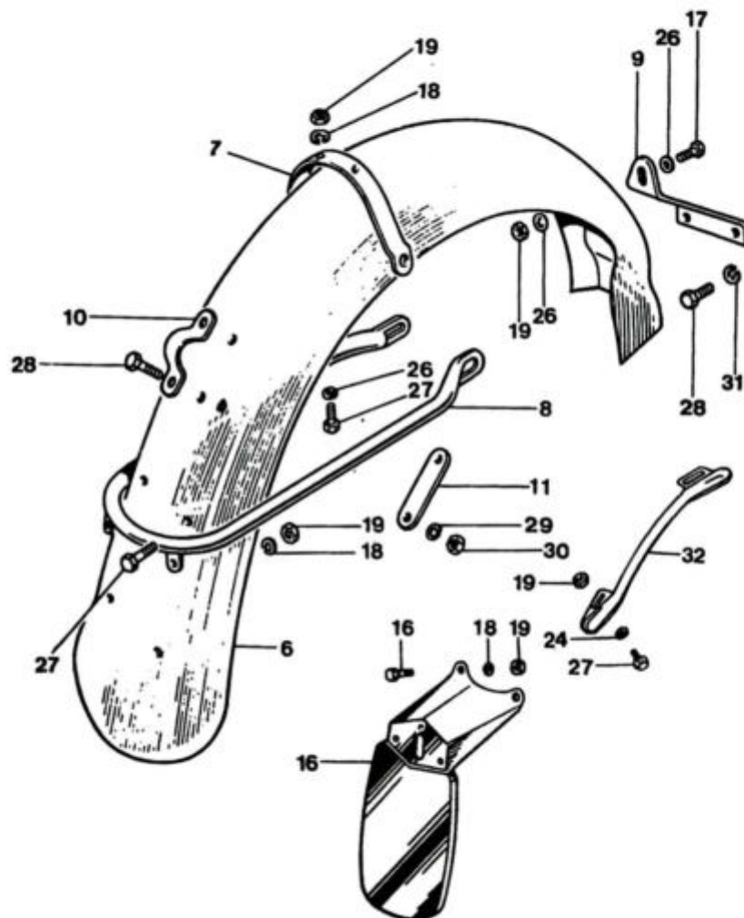
Fig. 25. MUDGUARDS
