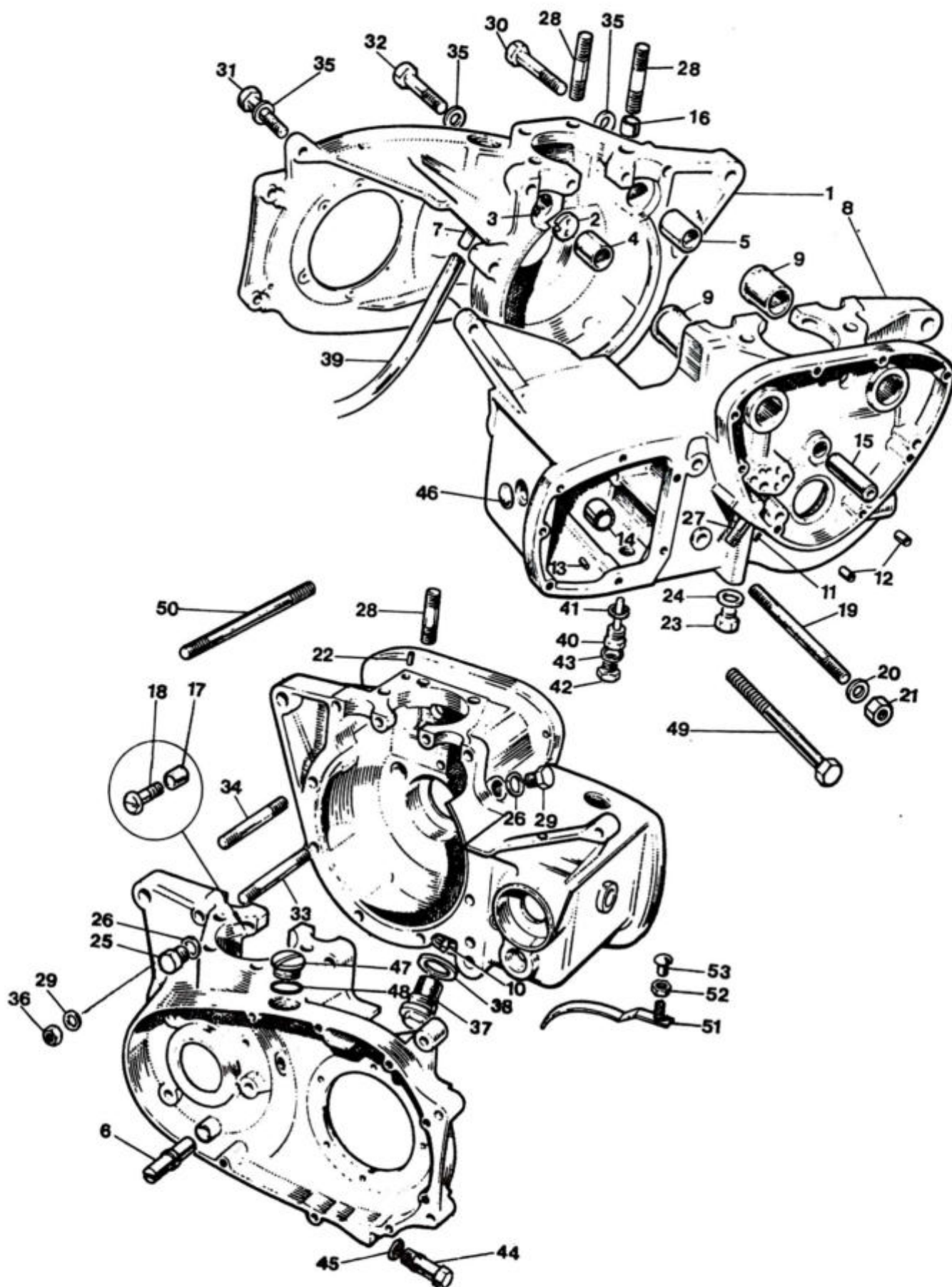
Fig. 2. CRANKCASE
