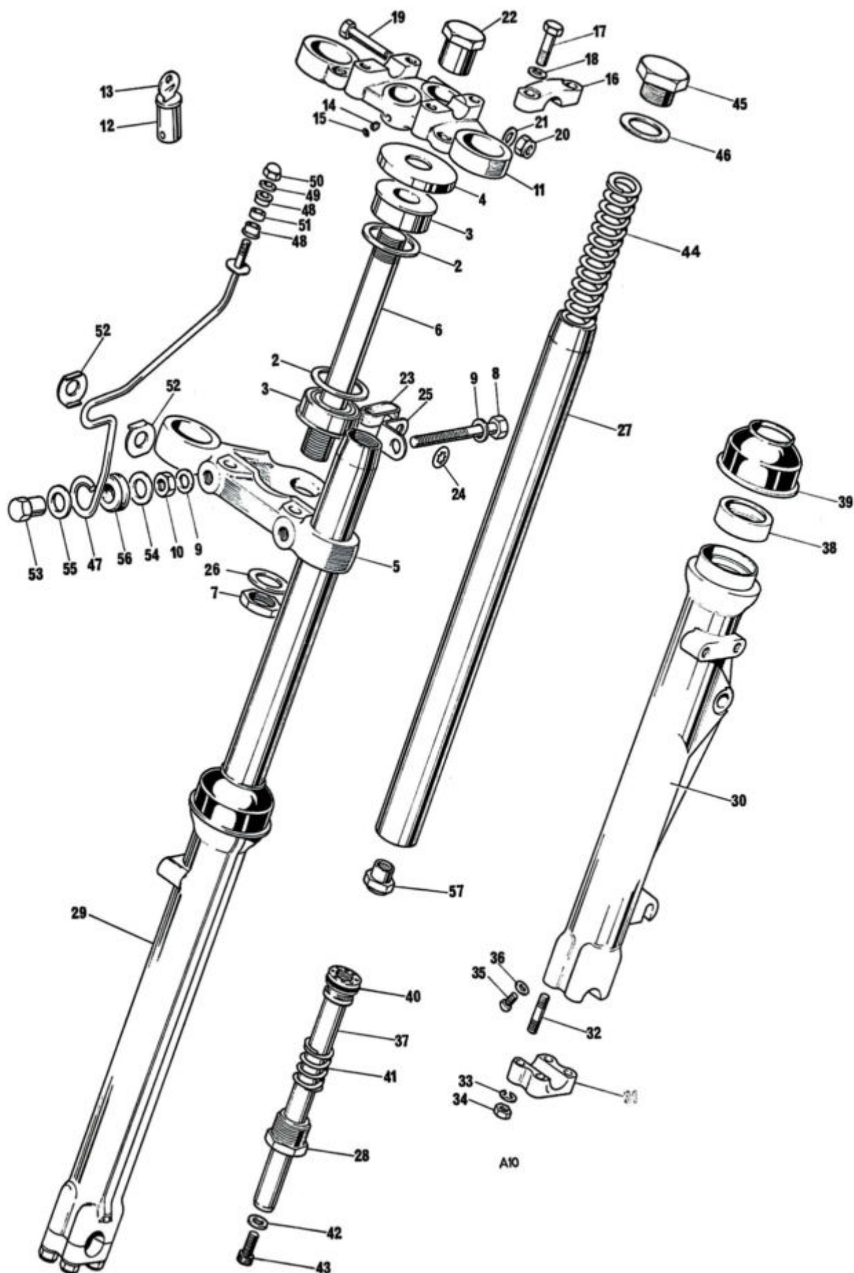
Fig. 10. TELESCOPIC FORKS
