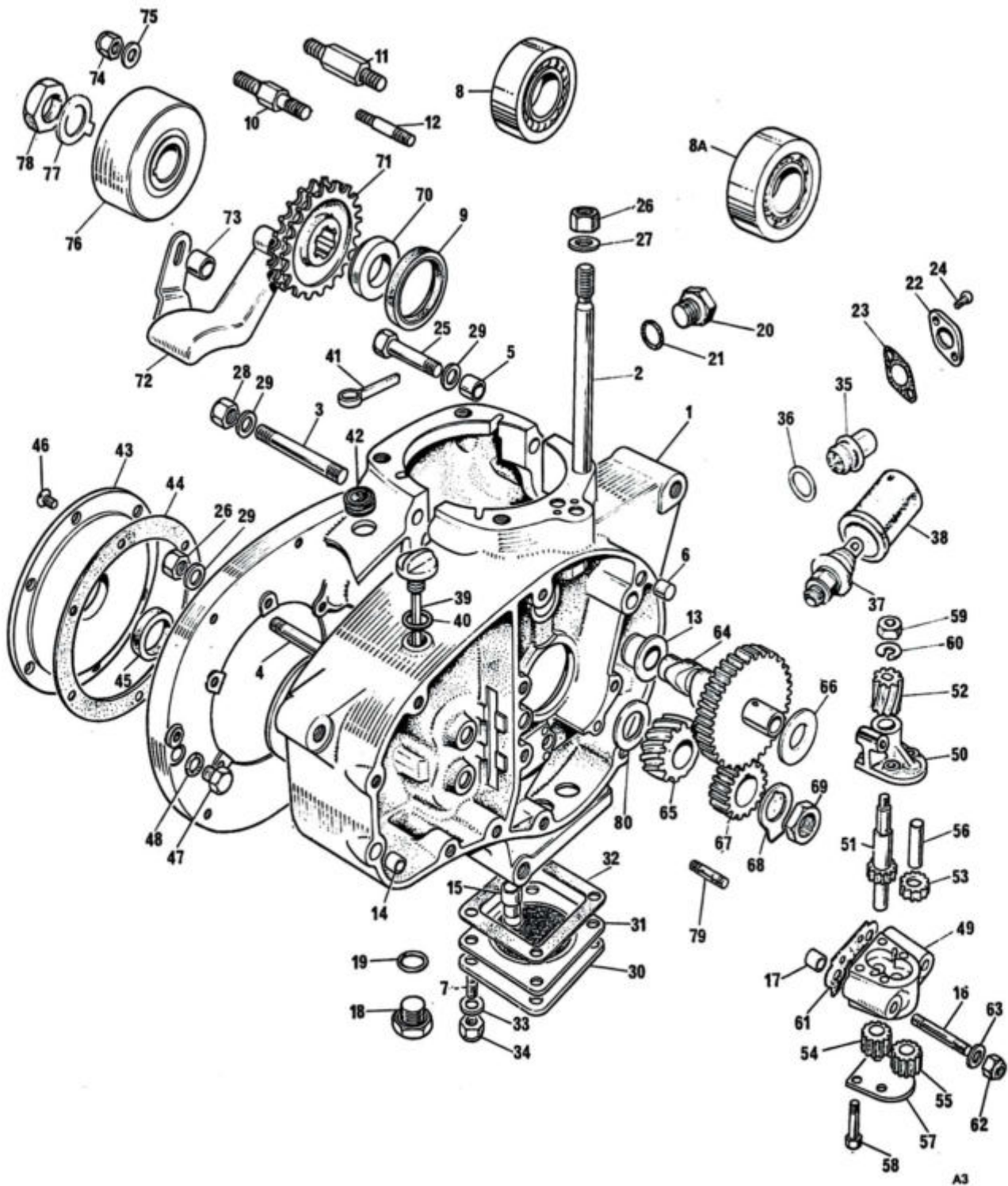
Fig. 3. CRANKCASE
