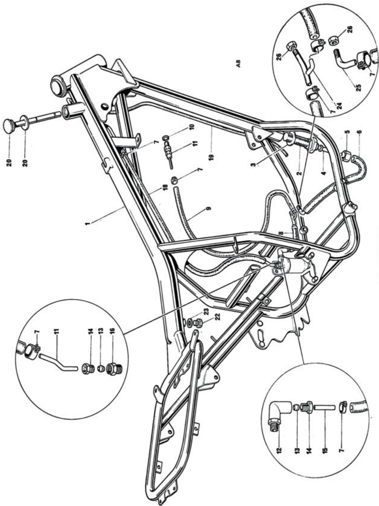
Fig. 8. FRAME
