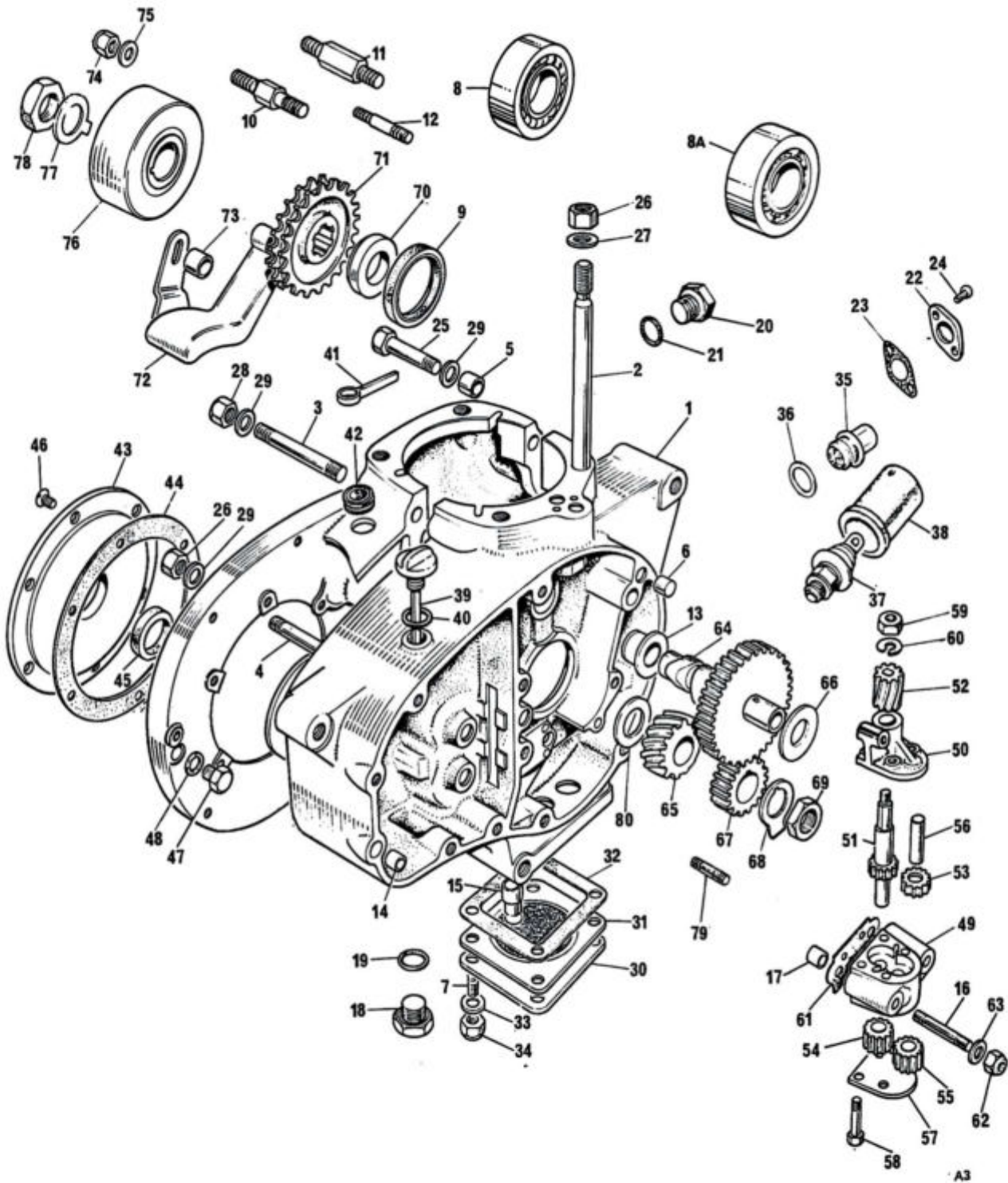
Fig. 3. CRANKCASE
