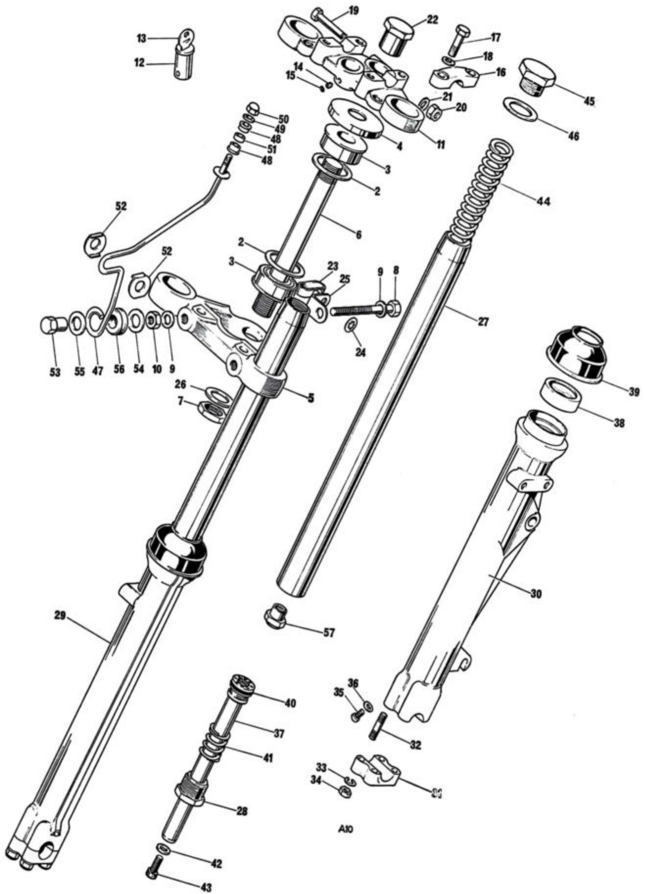
Fig. 10. TELESCOPIC FORKS
