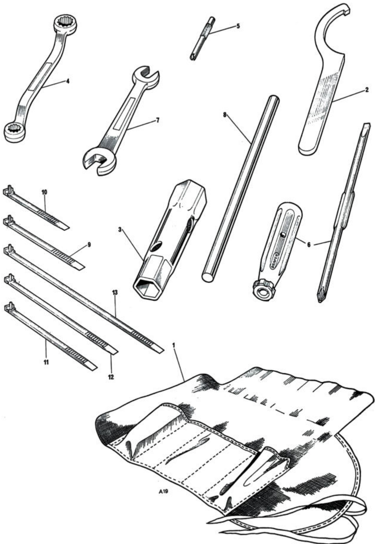
Fig. 19. TOOL KIT
