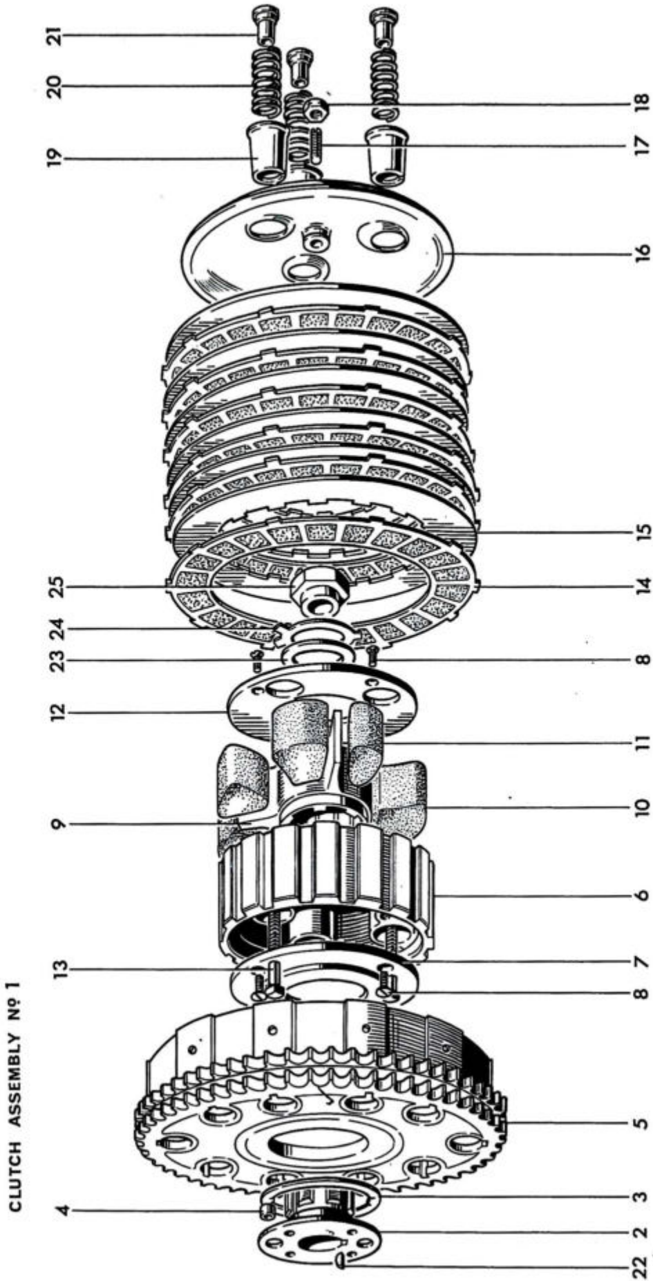
Fig. 9. CLUTCH
