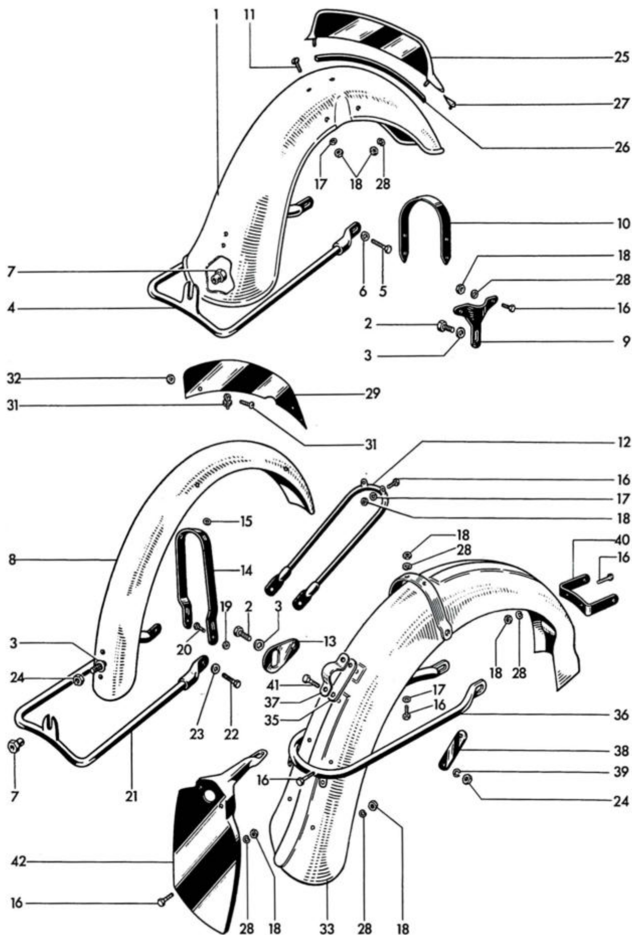
Fig. 20. MUDGUARDS
