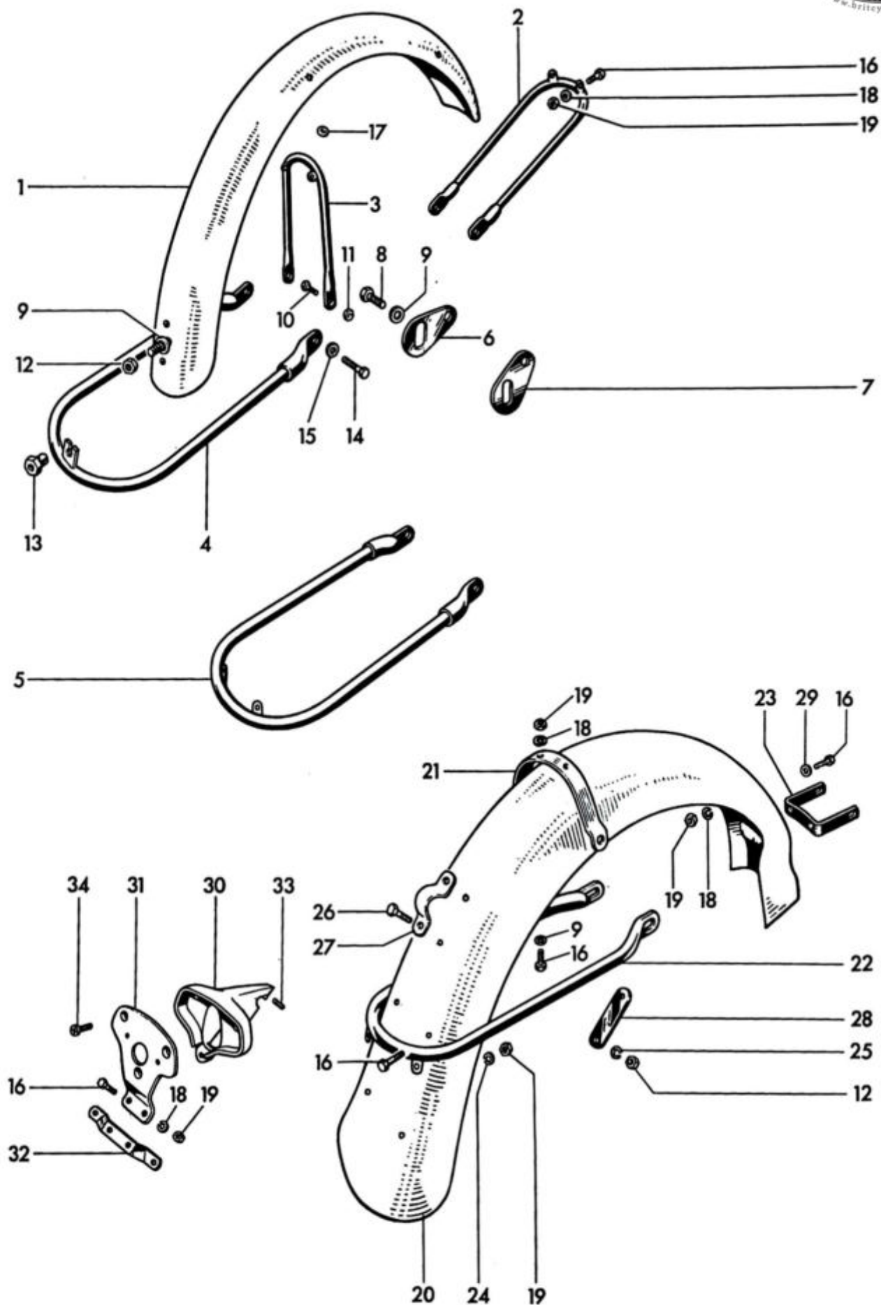
Fig. 23. FENDERS (U.S.A.)
