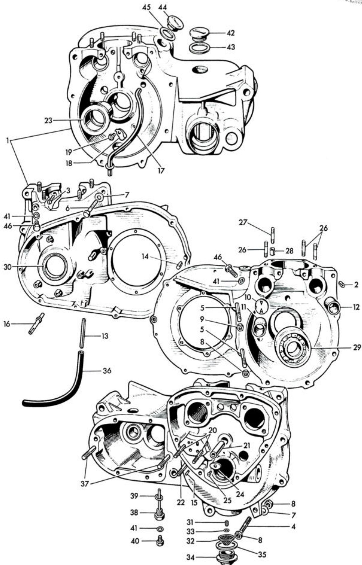
Fig. 2. CRANKCASE
