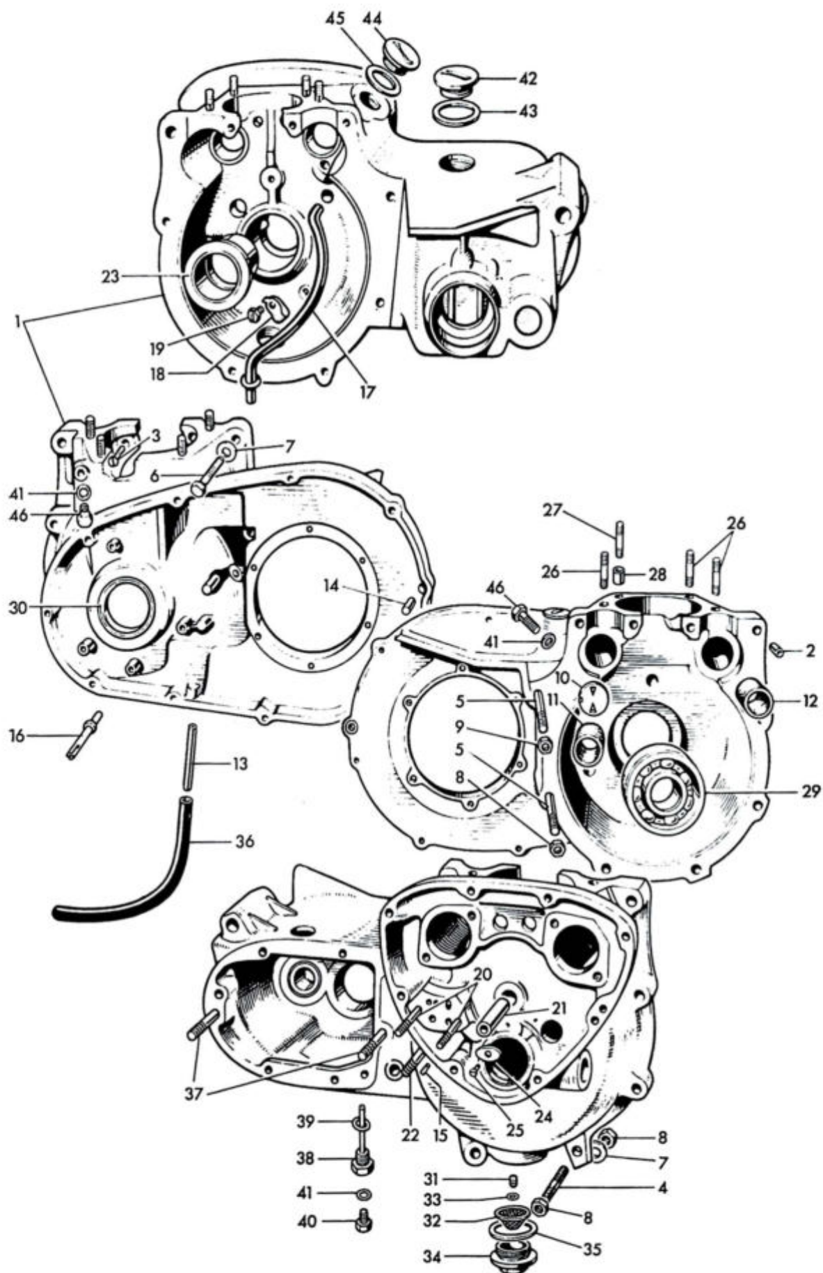
Fig. 2. CRANKCASE
