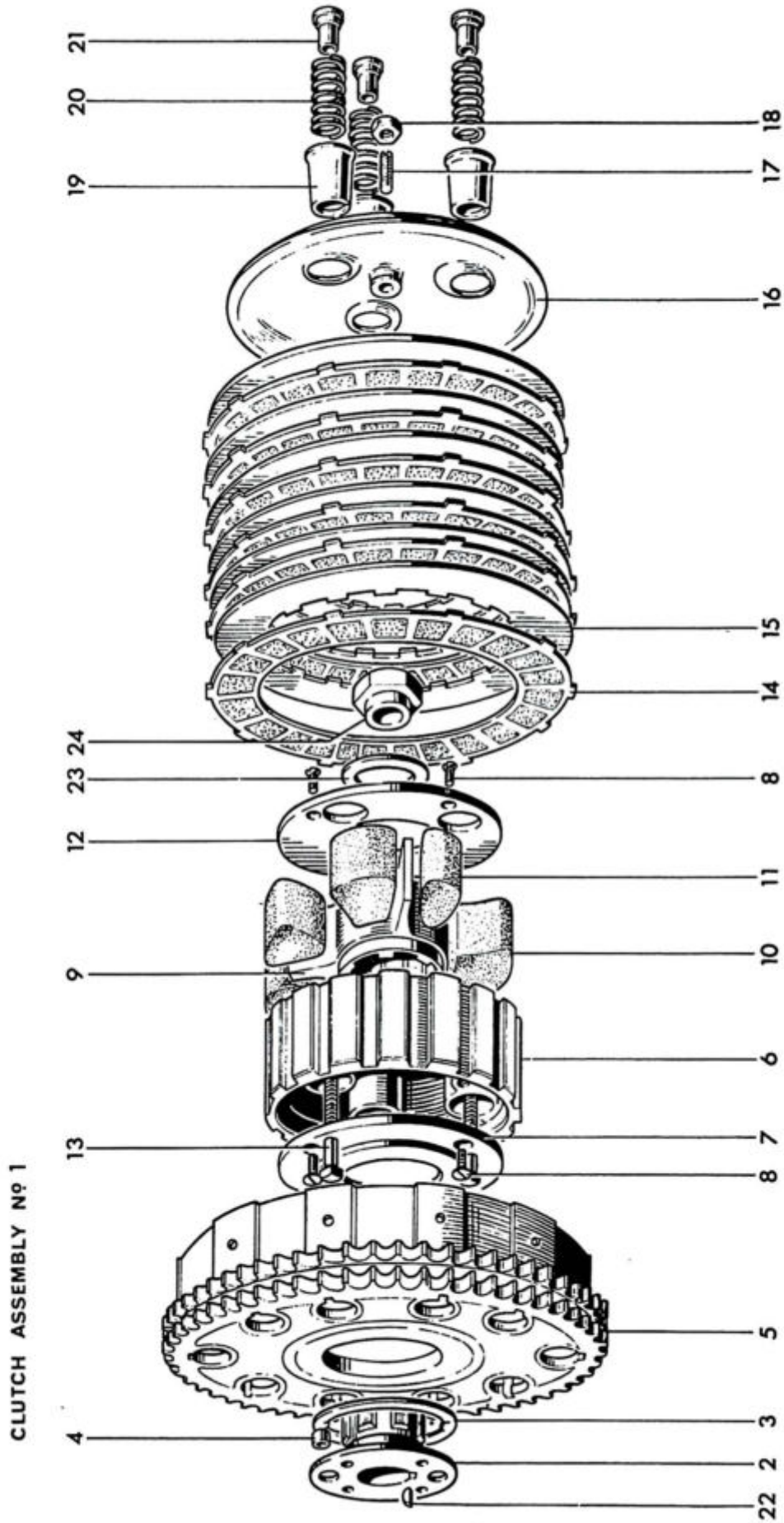
Fig. 11. CLUTCH
