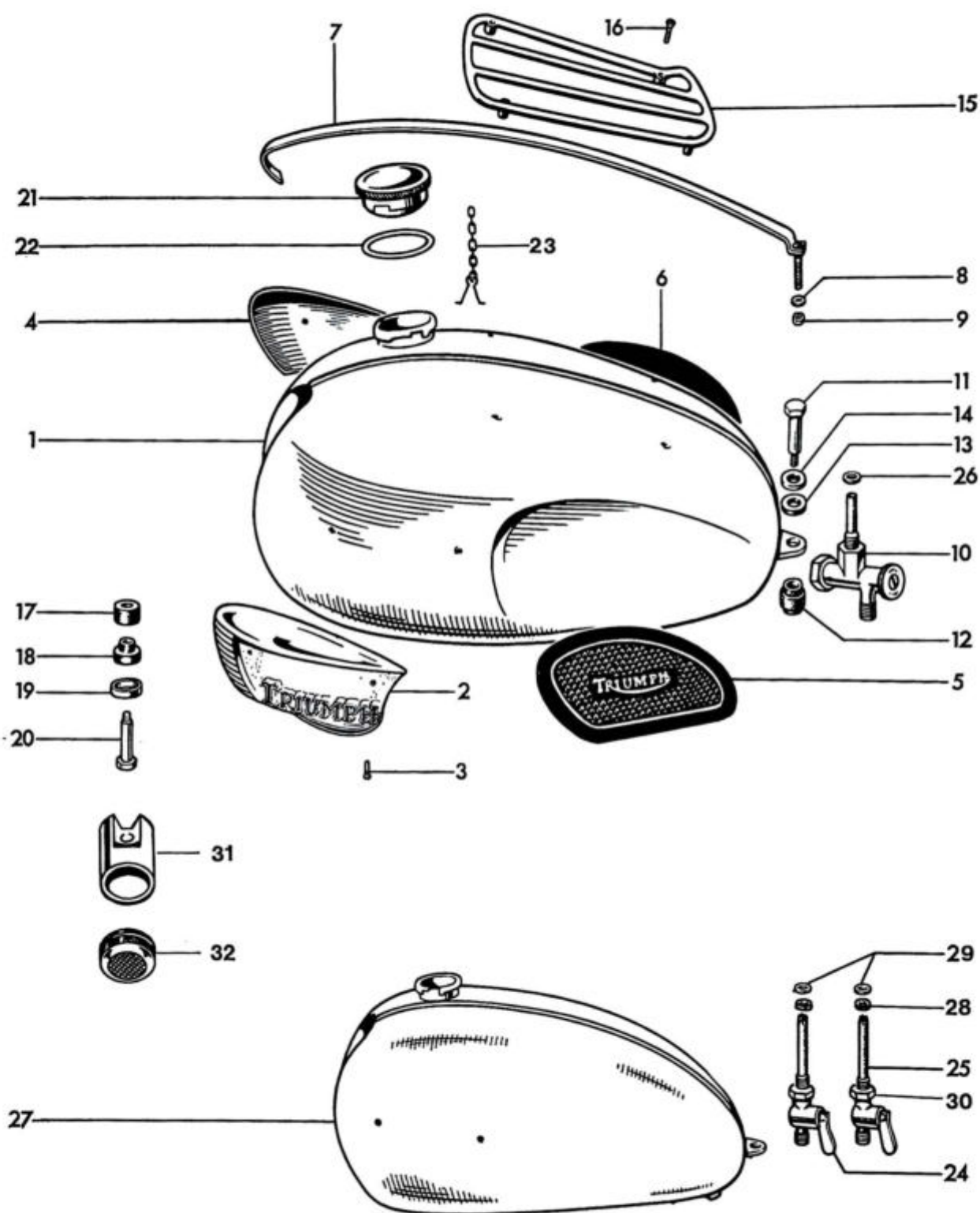
Fig. 24. PETROL TANK
