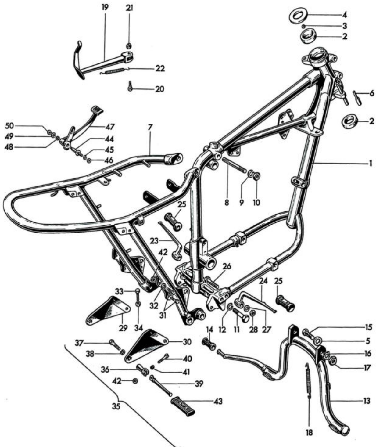
Fig. 15. FRAME
