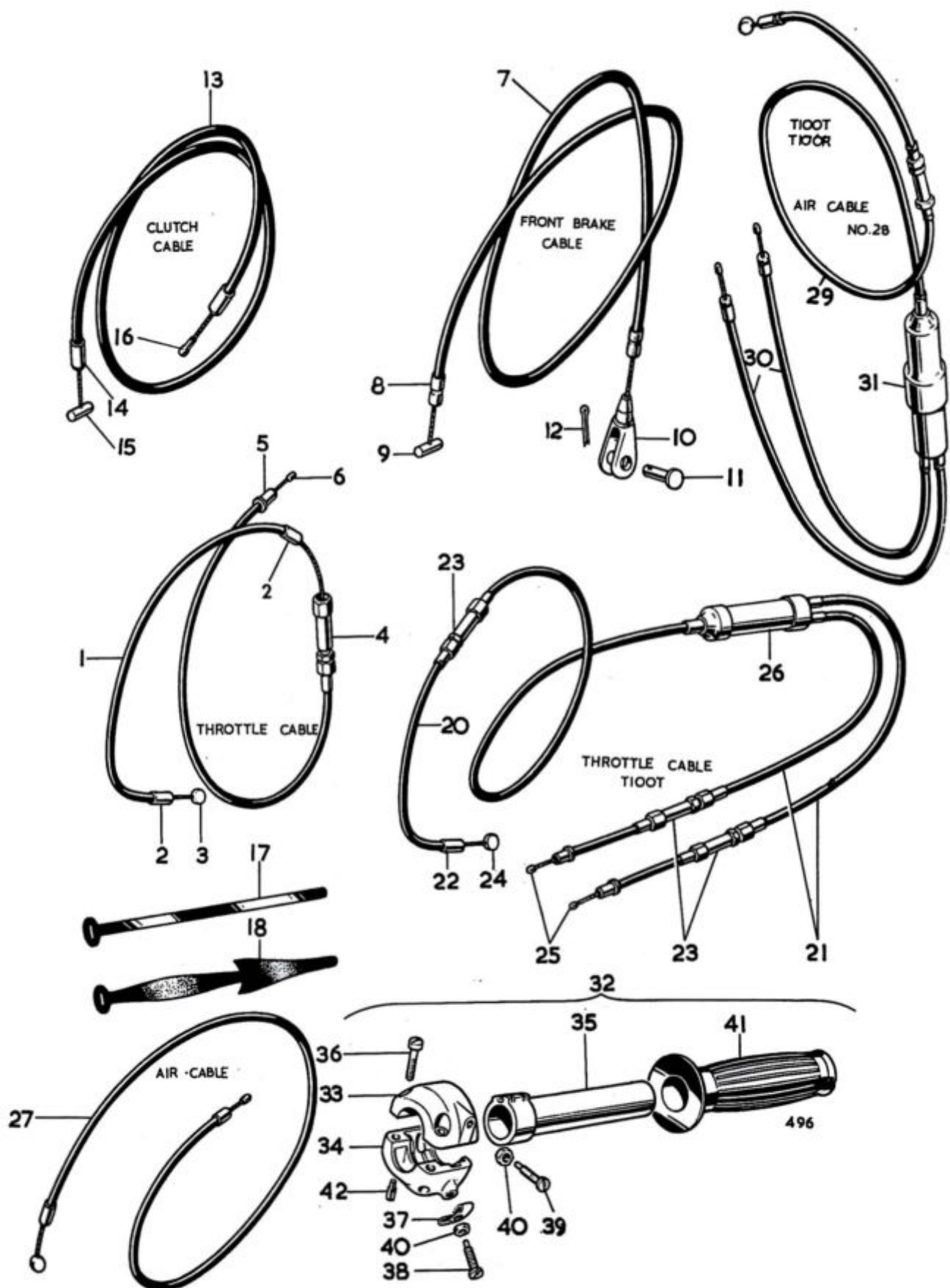
Fig. 28. CONTROL CABLES
