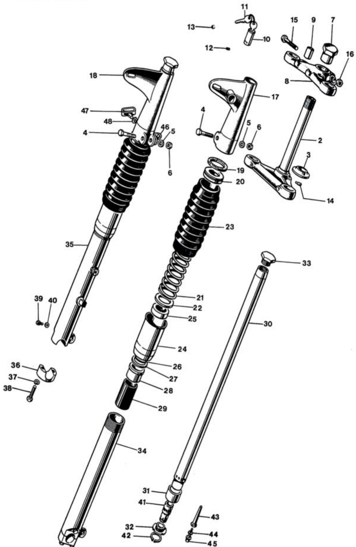
Fig. 17. TELESCOPIC FRONT FORK
