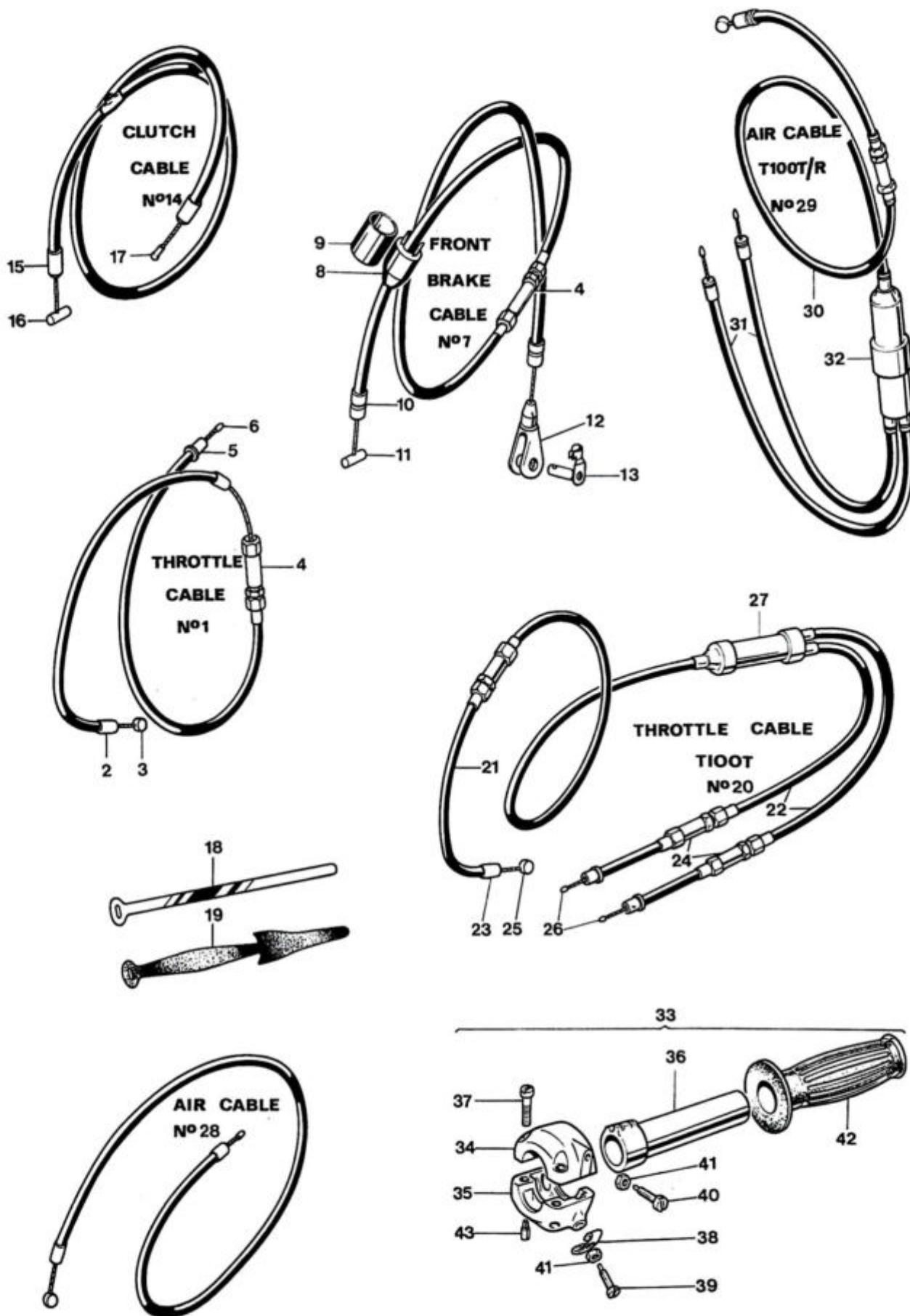
Fig. 29. CONTROL CABLES
