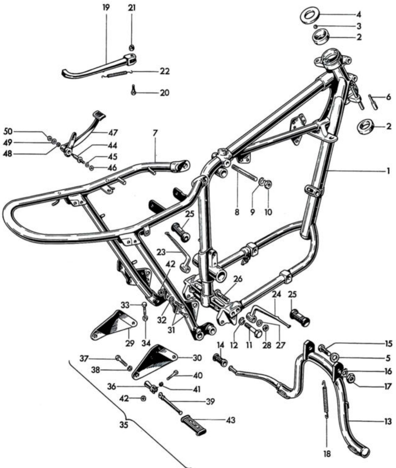
Fig. 15. FRAME
