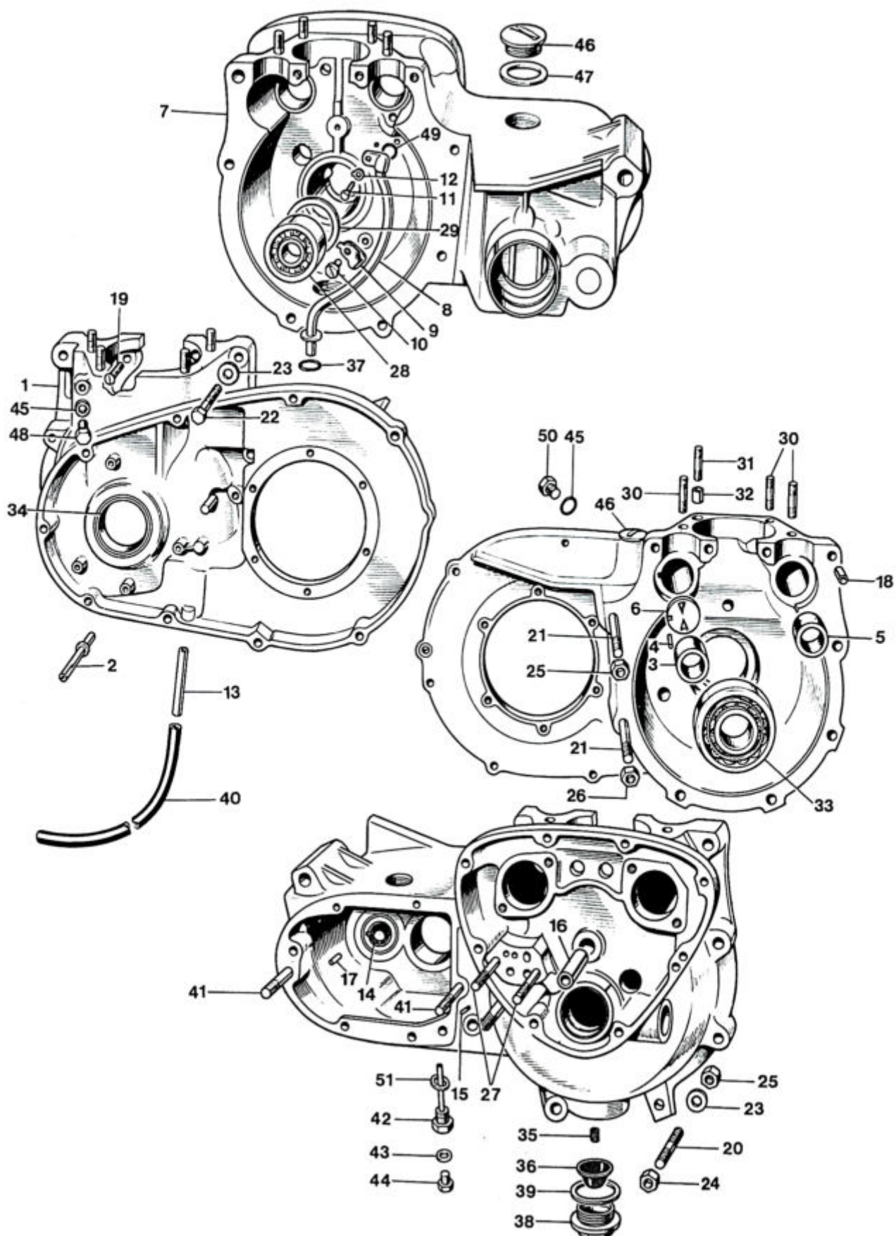
Fig. 2. CRANKCASE
