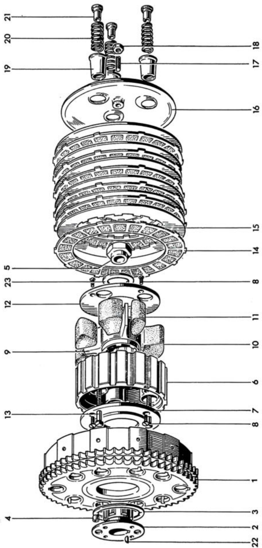
Fig. 11. CLUTCH
