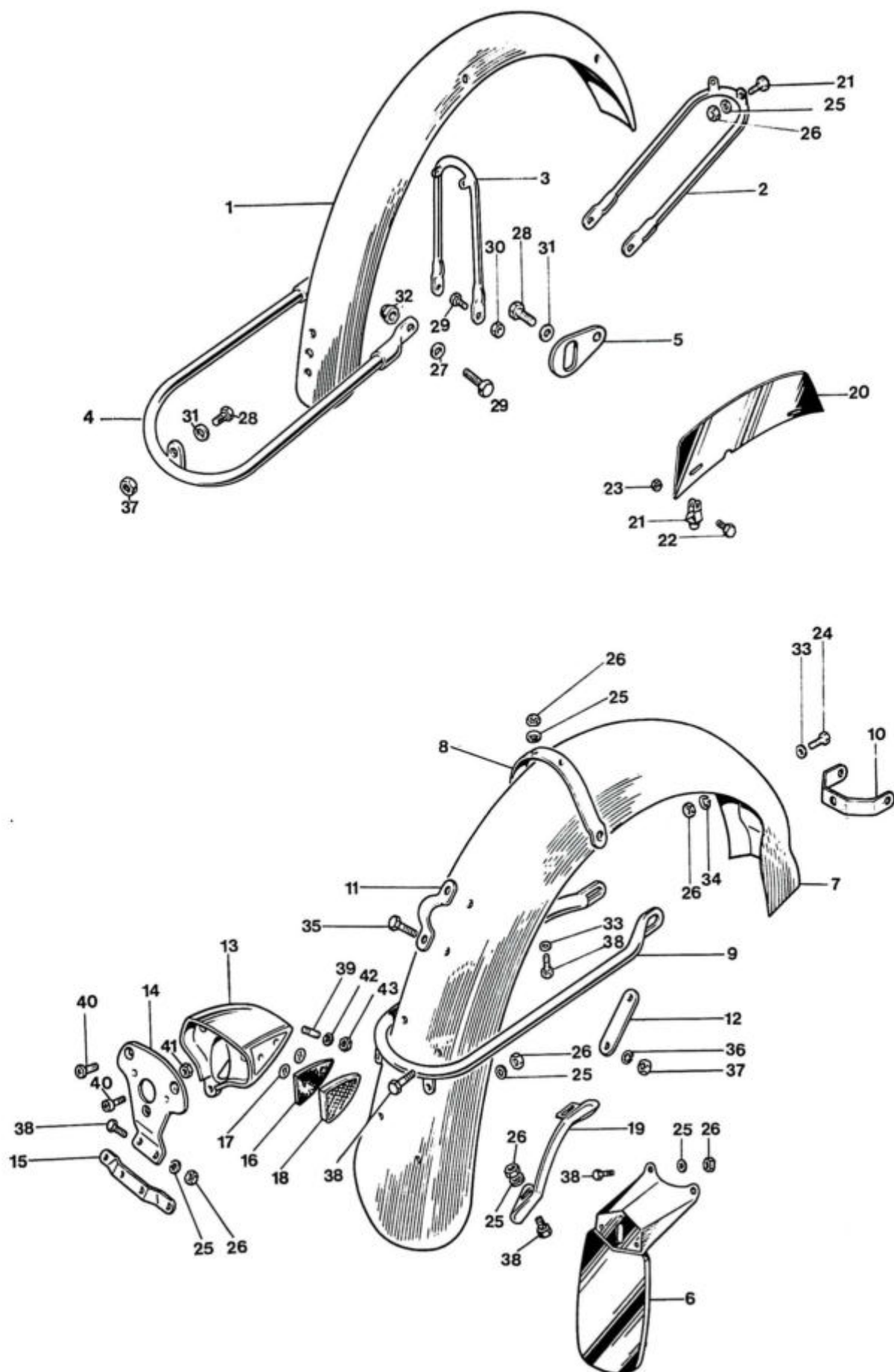
Fig. 23. MUDGUARDS (FENDERS U.S.A.)
