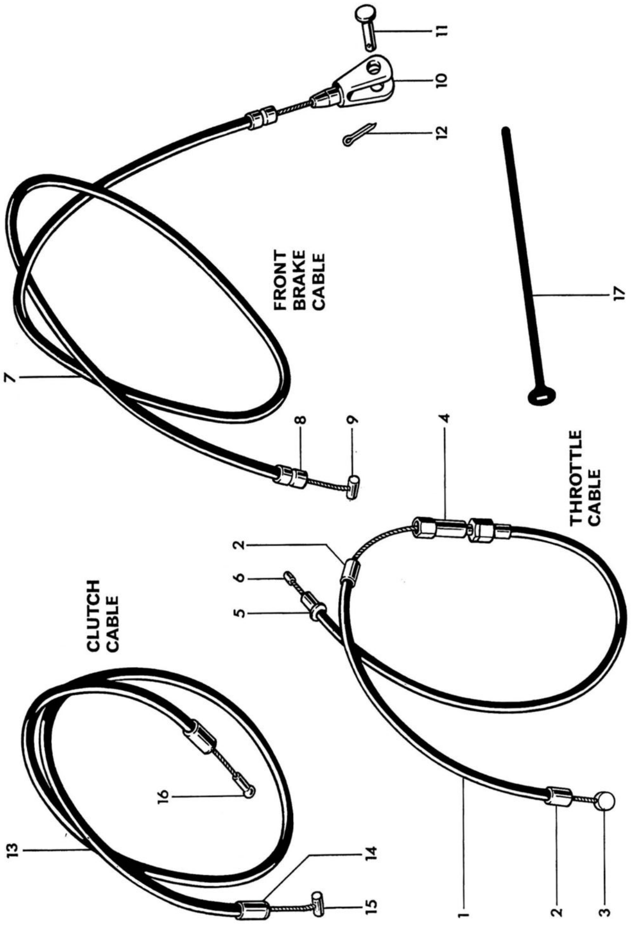
Fig. 26. CONTROL CABLES
