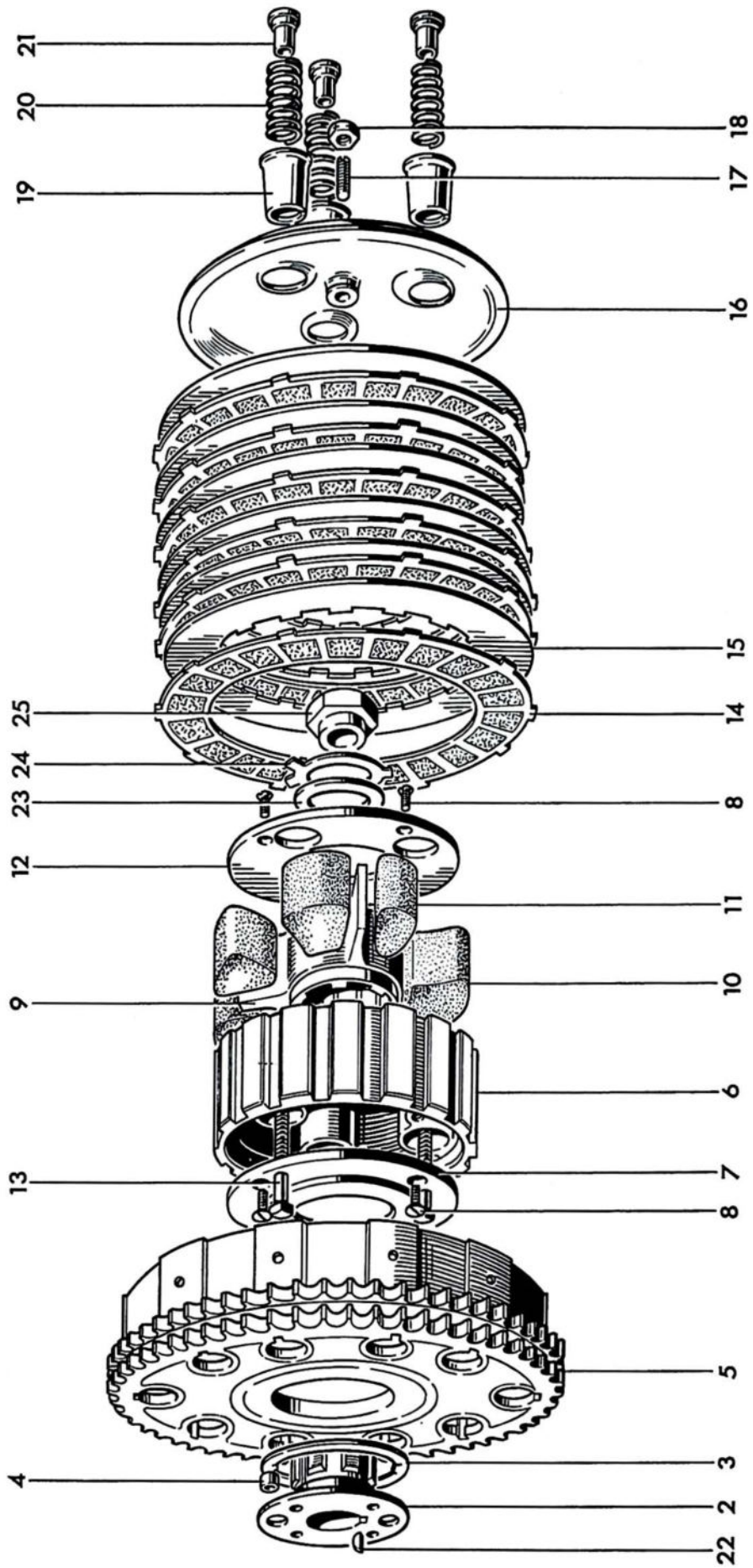
Fig. 9. CLUTCH
