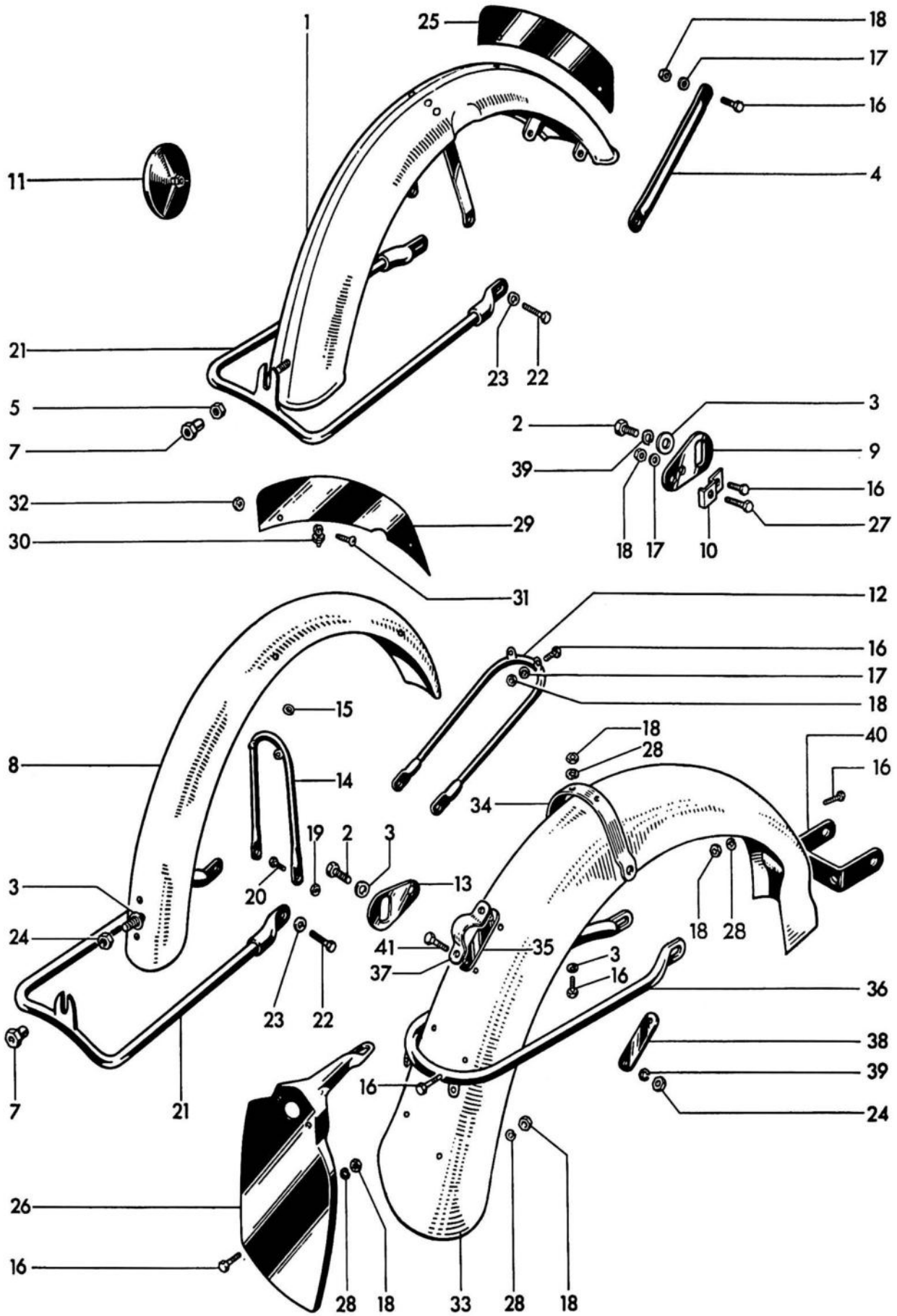
Fig. 20. MUDGUARDS
