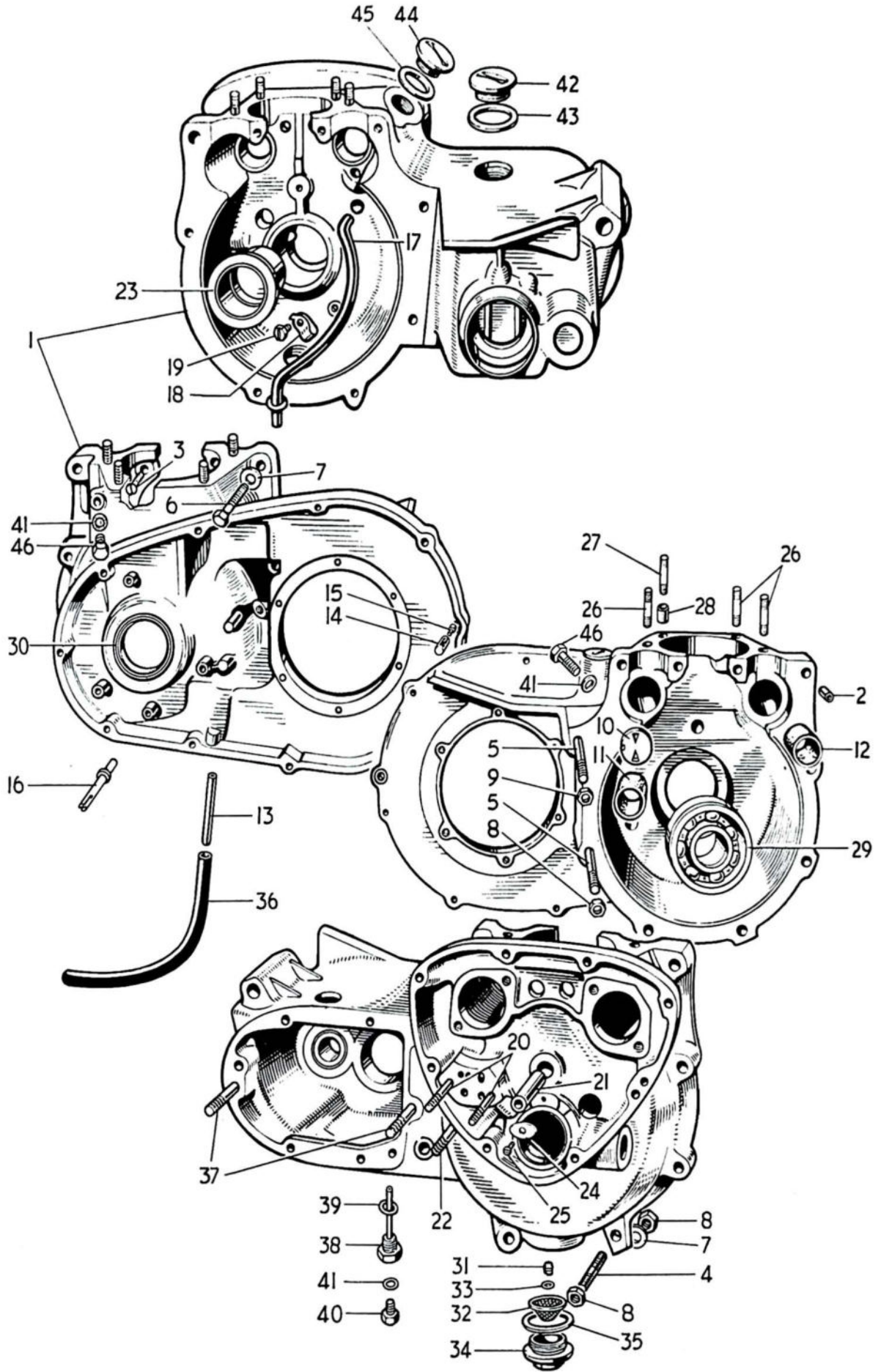
Fig. 2. CRANKCASE
