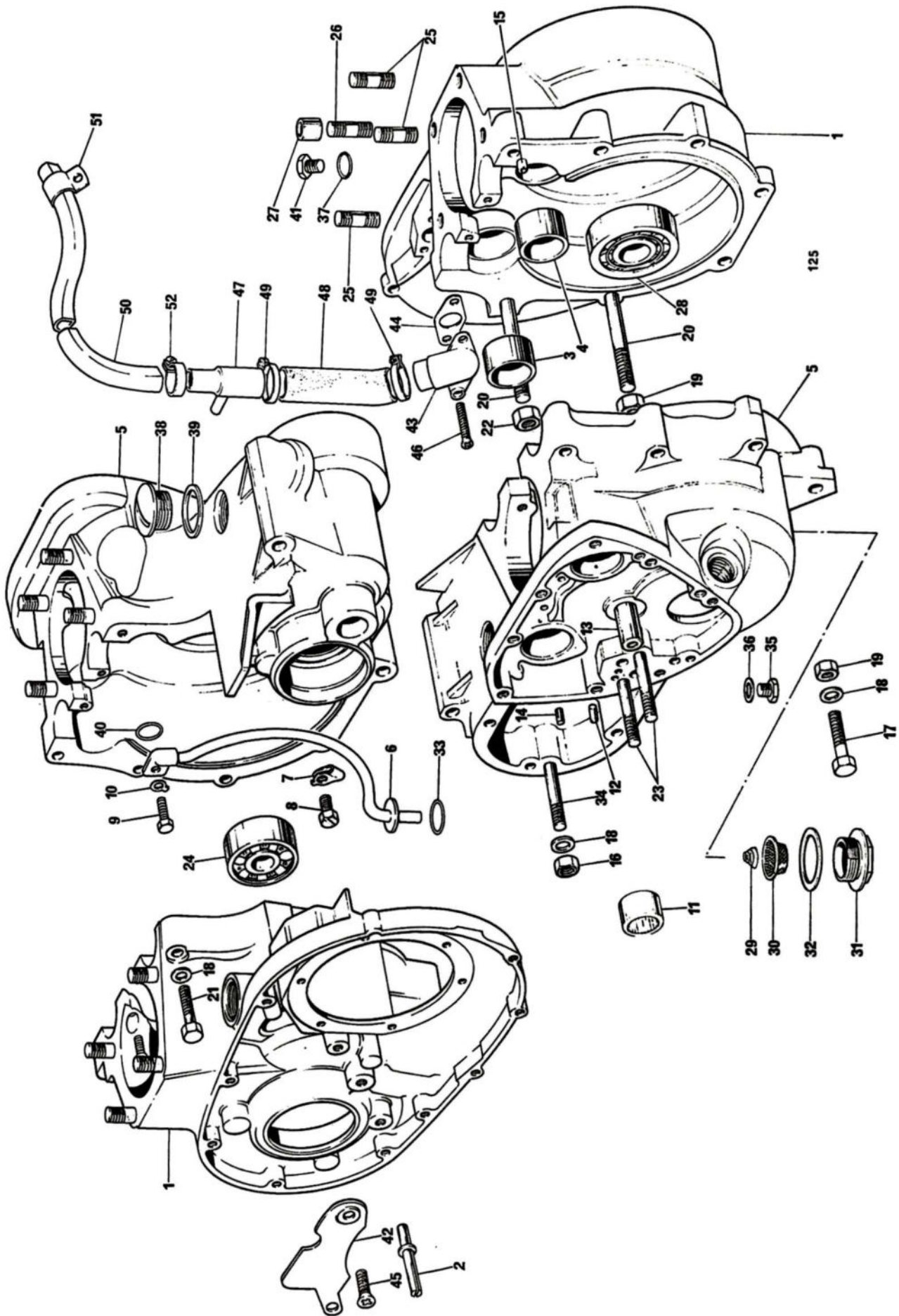
Fig. 2. CRANKCASE
