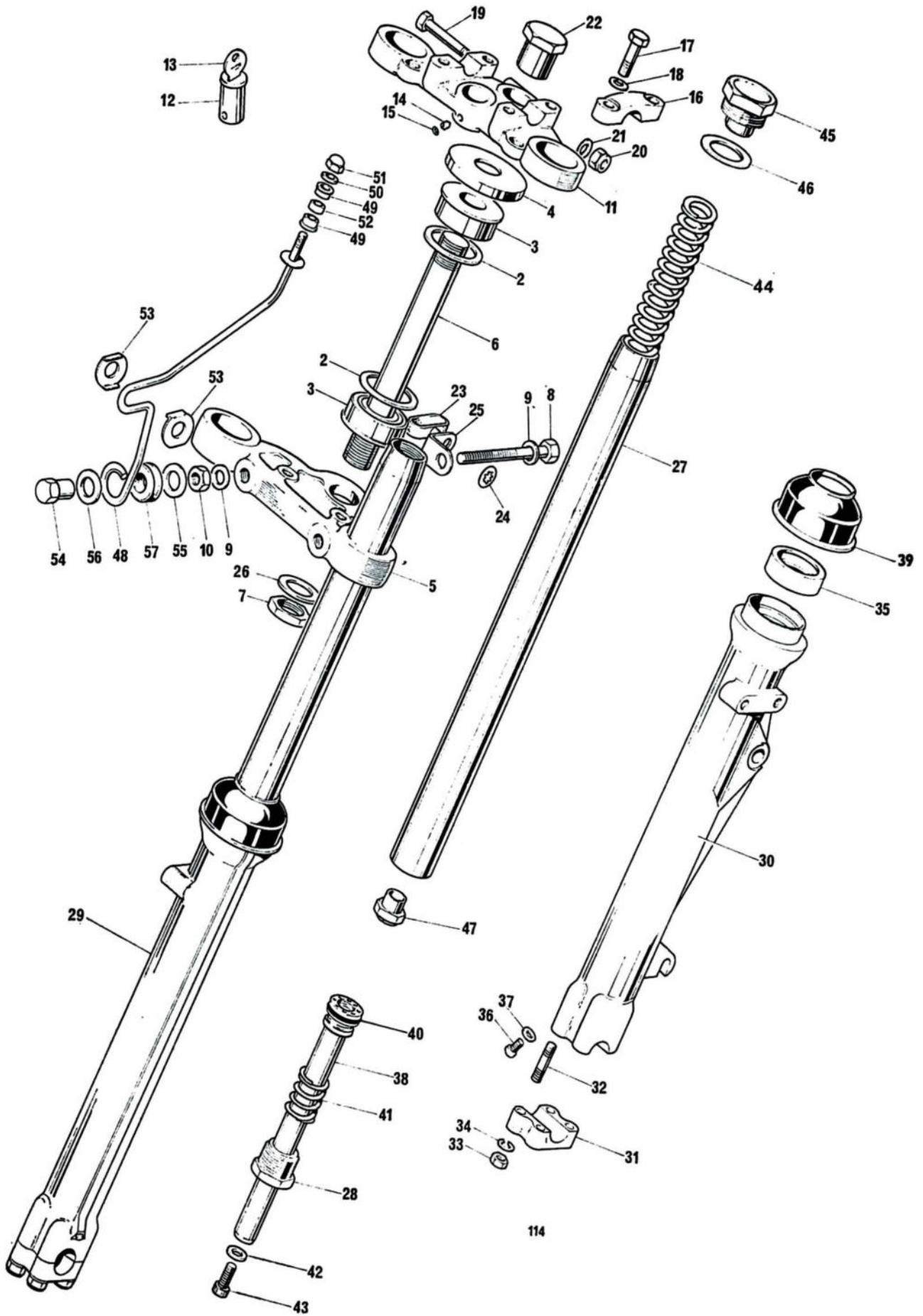
Fig. 15. TELESCOPIC FORKS
