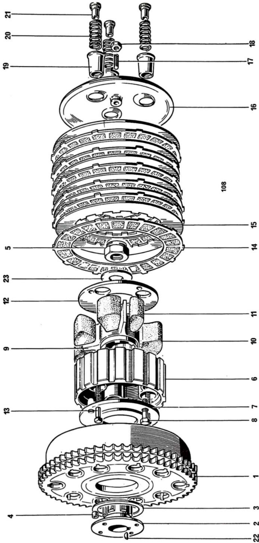
Fig. 9. CLUTCH
