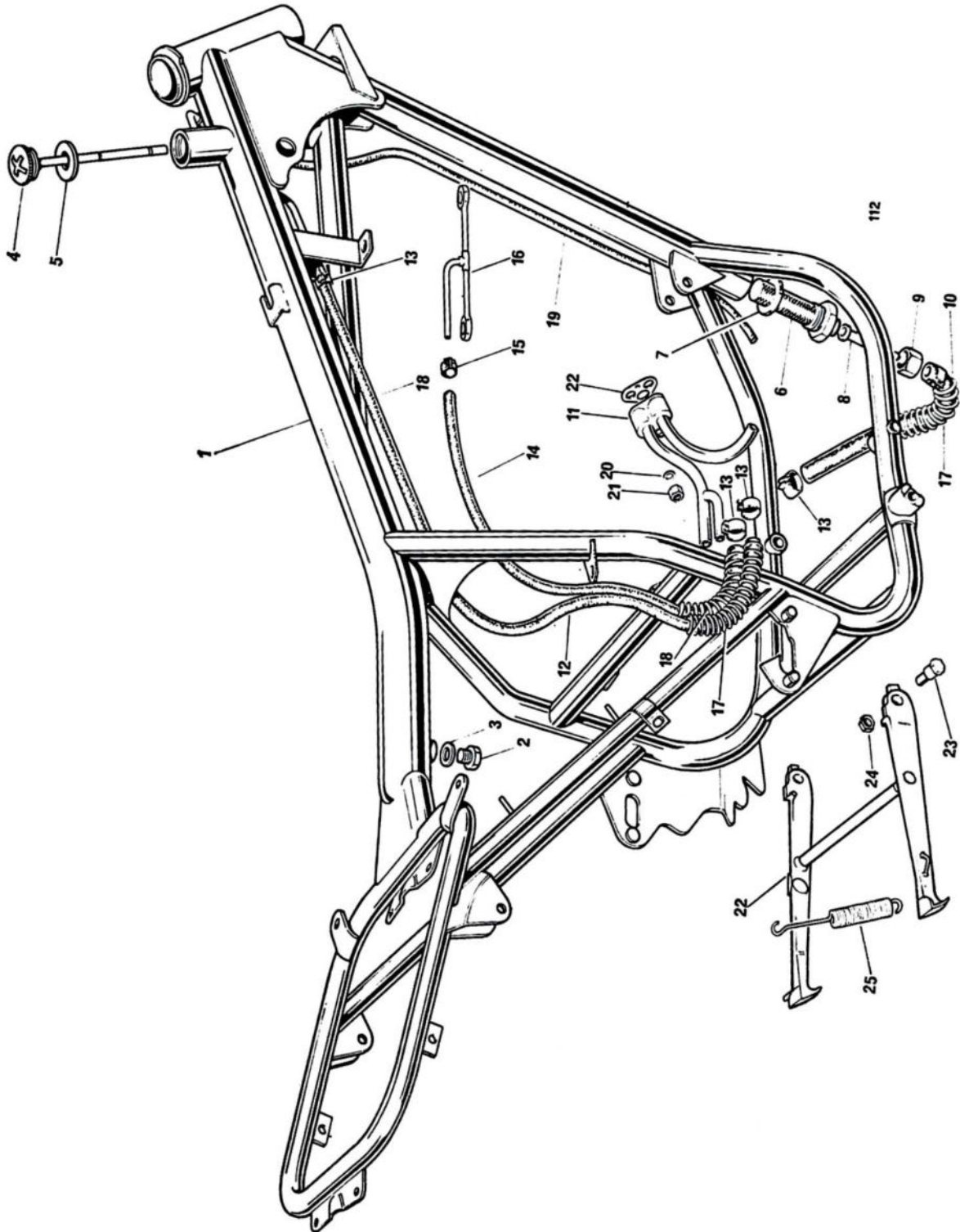
Fig. 13. FRAME
