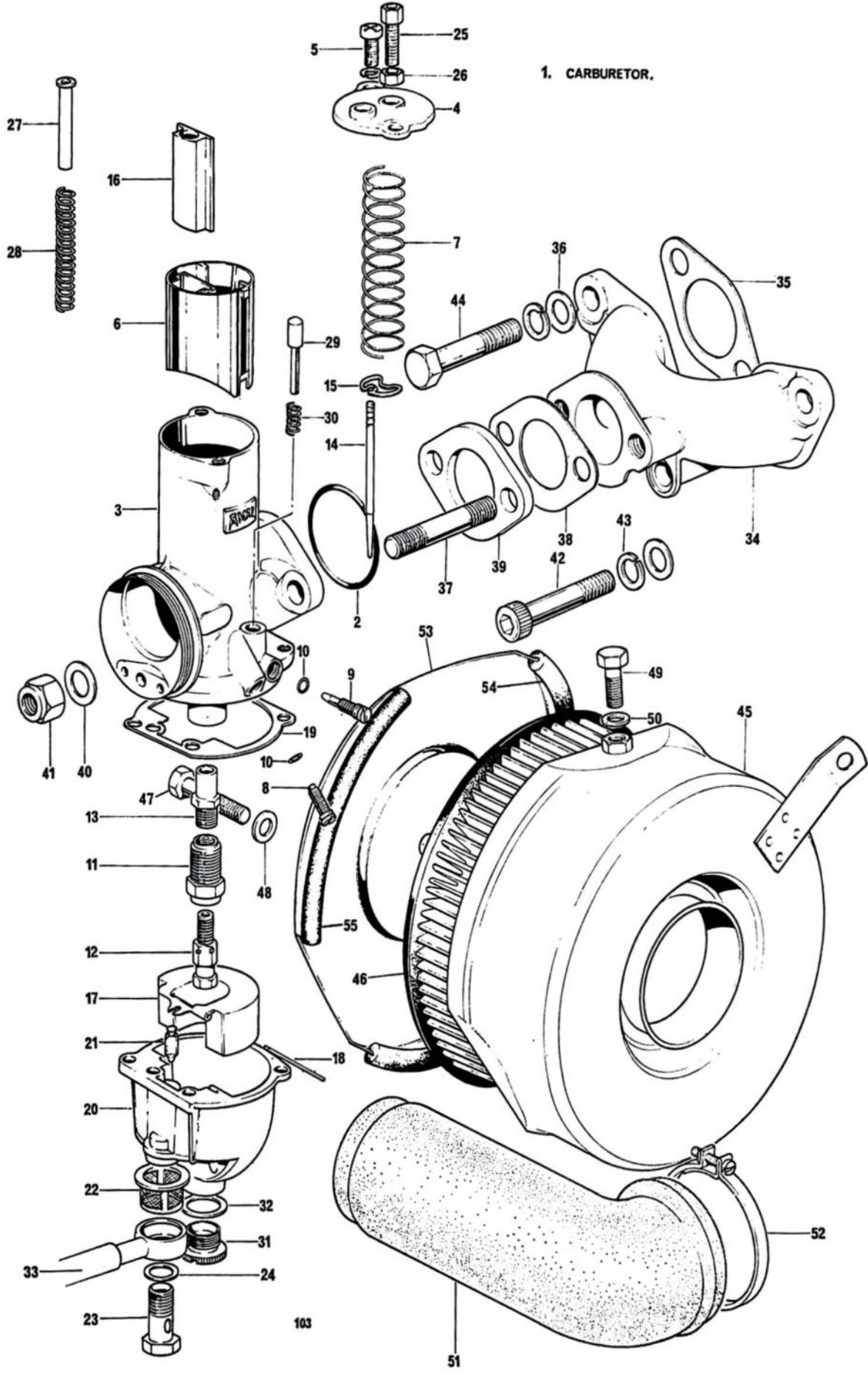
Fig. 4. CARBURETOR
