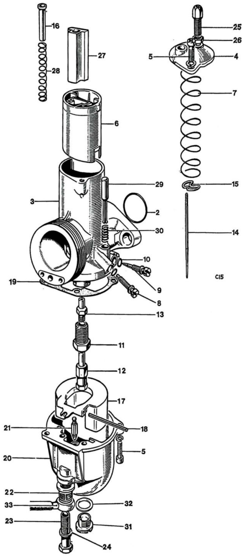
Fig. 4. CARBURETOR
