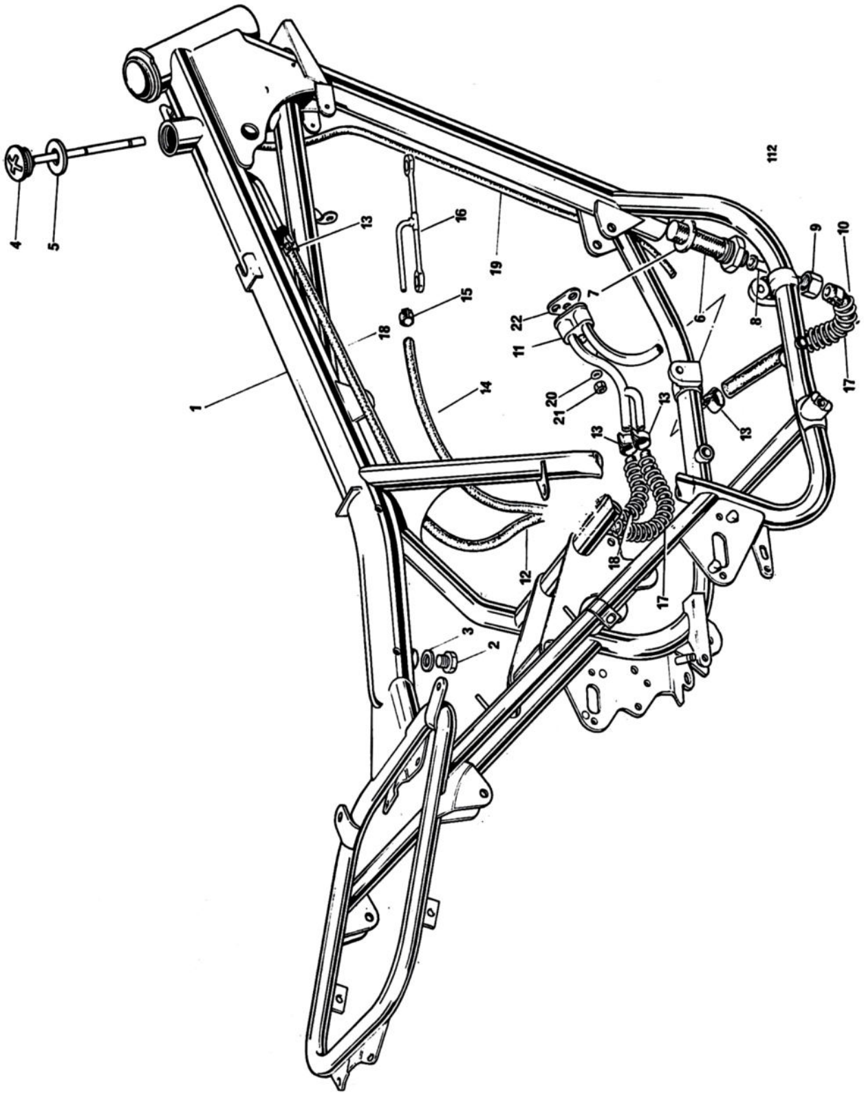
Fig. 14. FRAME
