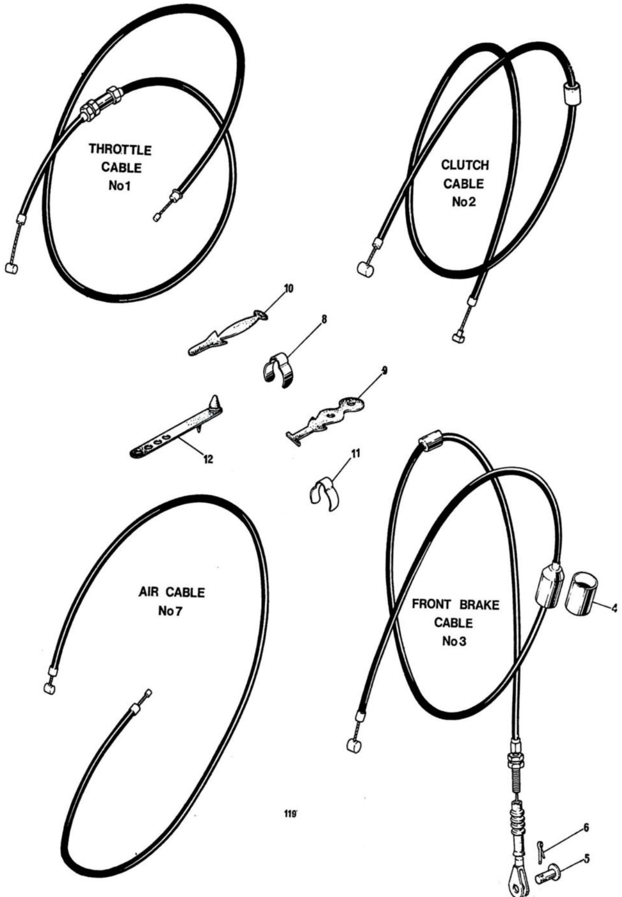
Fig. 21. CONTROL CABLES
