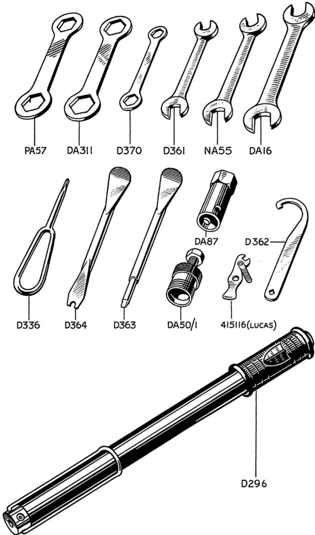
FIG. 15 TOOLKIT
