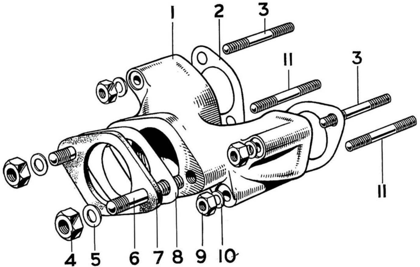
FIG. I INLET MANIFOLD
